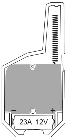
Рис.1. Радиокнопка со снятой задней крышкой
