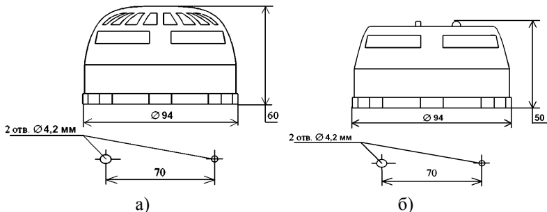
Рисунок 1. Габаритные и установочные размеры извещателей:
