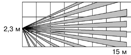
Рисунок 2 – Диаграмма зоны обнаружения извещателя «Фотон-12Б-РК»
