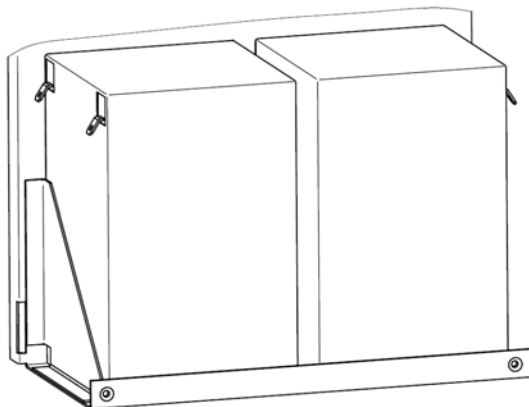
Рисунок 2. Ориентация батарей в случае установки двух АКБ.
