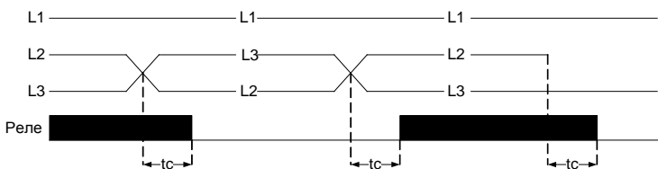
Рисунок 4. Контроль порядка чередования и обрыва фаз
