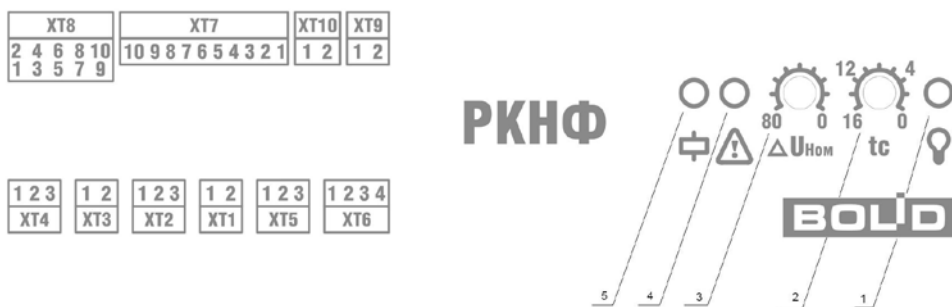
Рисунок 3. Лицевая панель РКНФ
