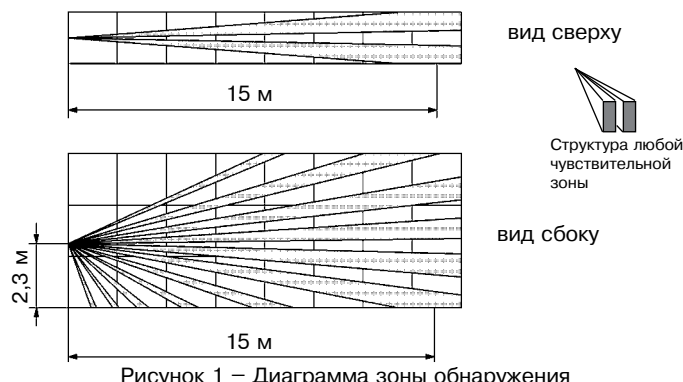
Рисунок 1 – Диаграмма зоны обнаружения
