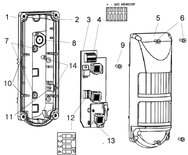
Рисунок 2 - Конструкция извещателя
