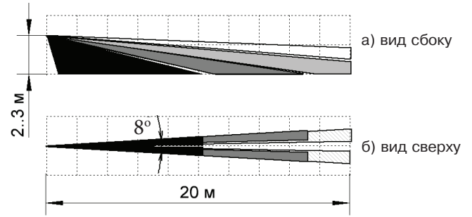
Рисунок 1 - Диаграмма зоны обнаружения извещателя
