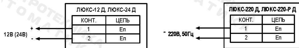
Рис.1. Схемы подключения.
