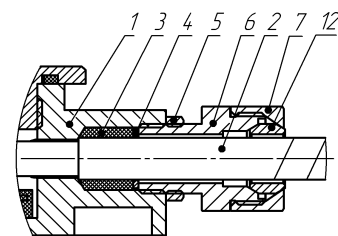
в) монтаж бронированным кабелем в кабельном вводе КВВ17
