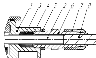
а) монтаж бронированным кабелем в кабельном вводе КВВ12
