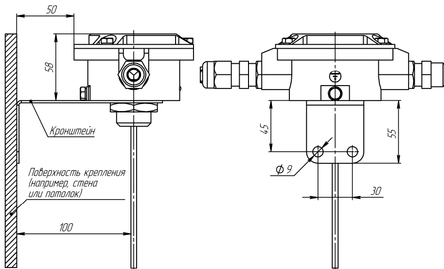
Рисунок 2. Пример крепления извещателя с помощью кронштейна.
