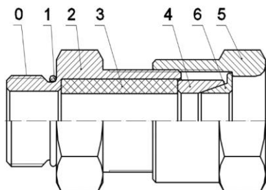
KB5 – для монтажа бронированного кабеля
