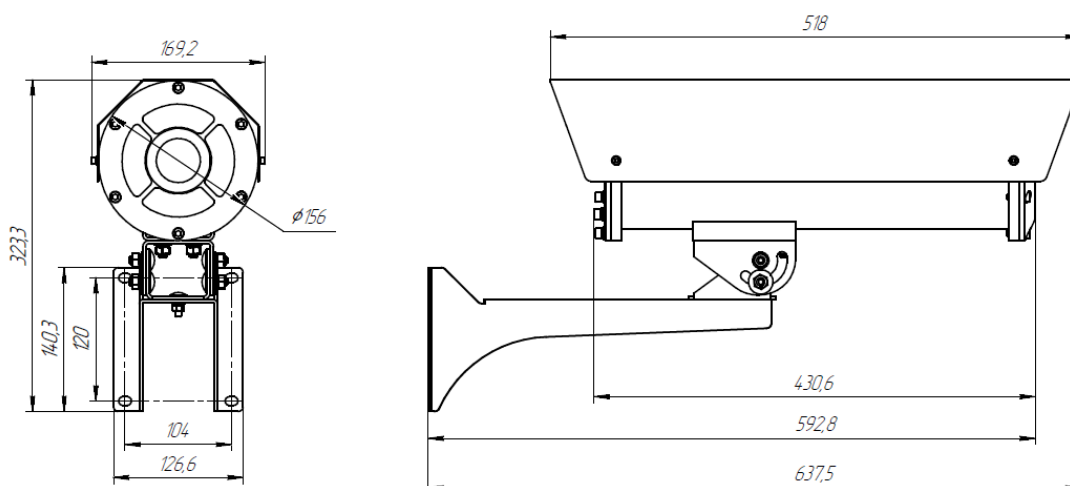
Рисунок 4.2 – Габаритные размеры термокожуха (мм)
