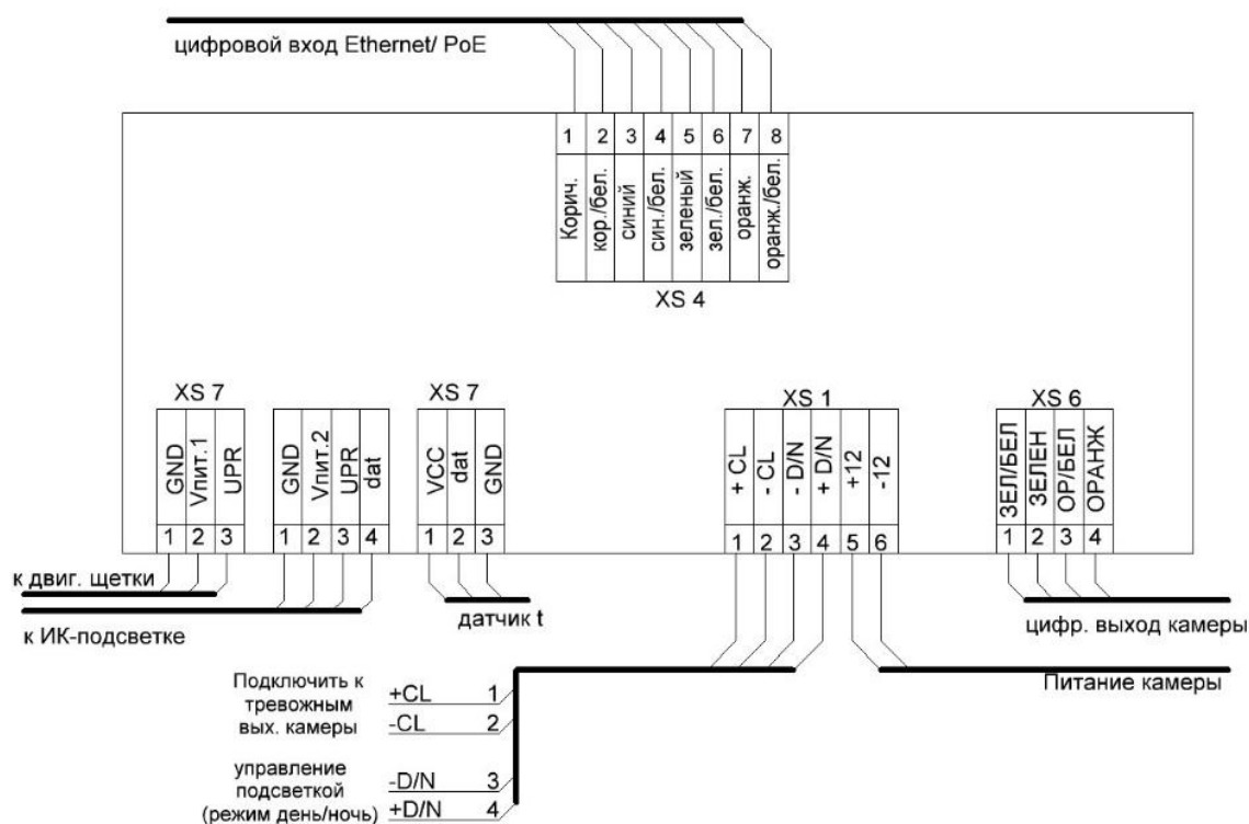
Рисунок 4.8 – Схема подключения термокожуха с напряжением питания по PoE
