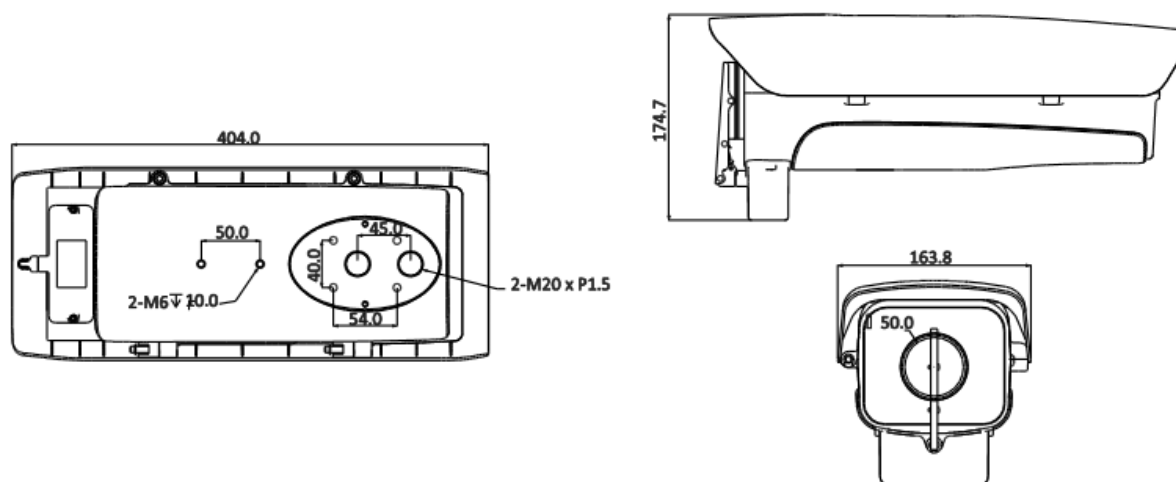
Рисунок 4.1 – Габаритные размеры
