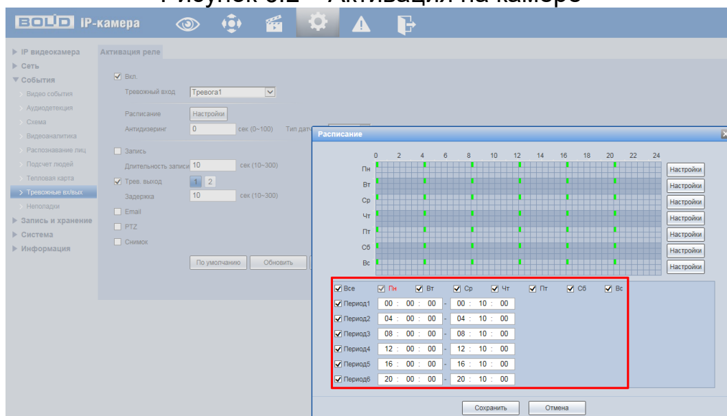
Рисунок 6.3 – Расписание включения
