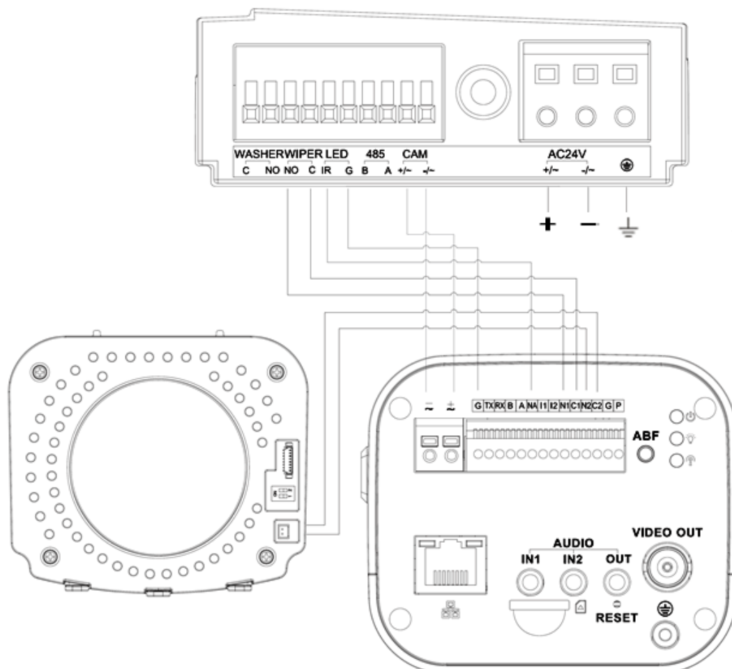
Рисунок 6.1 – Схема подключения
