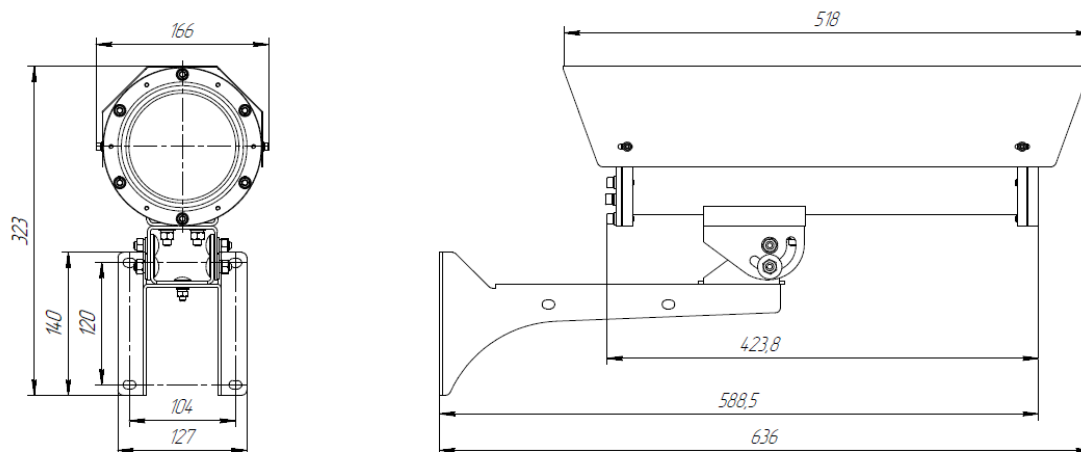
Рисунок 4.2 – Габаритные размеры термокожуха (мм)
