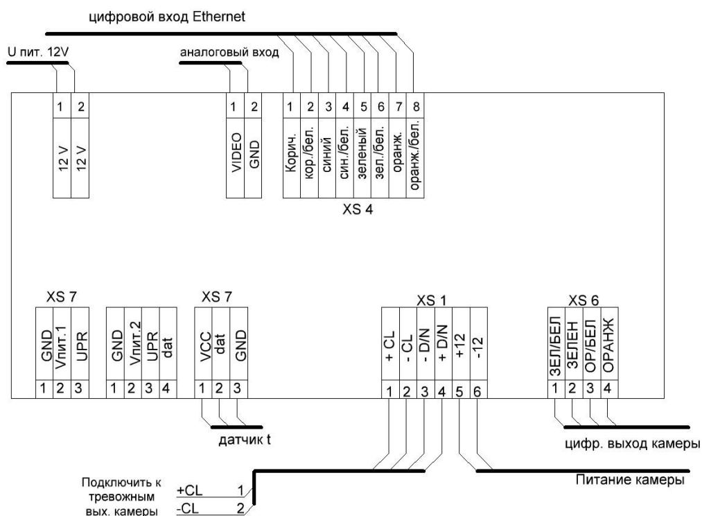
Рисунок 4.4 – Схема подключения термокожуха с напряжением
