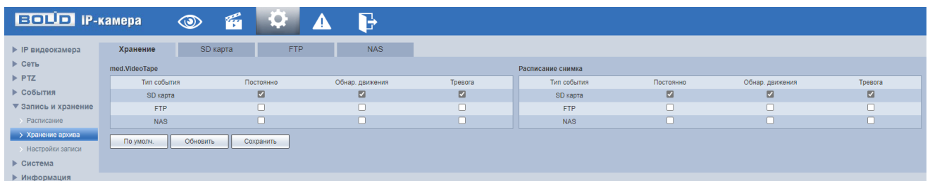
Рисунок 9.118 – Вкладка «Хранение»
