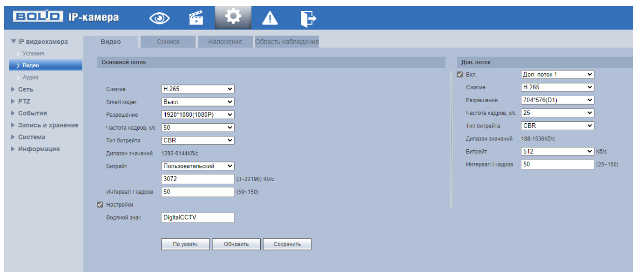
Рисунок 9.36 – Вкладка «Видео»
