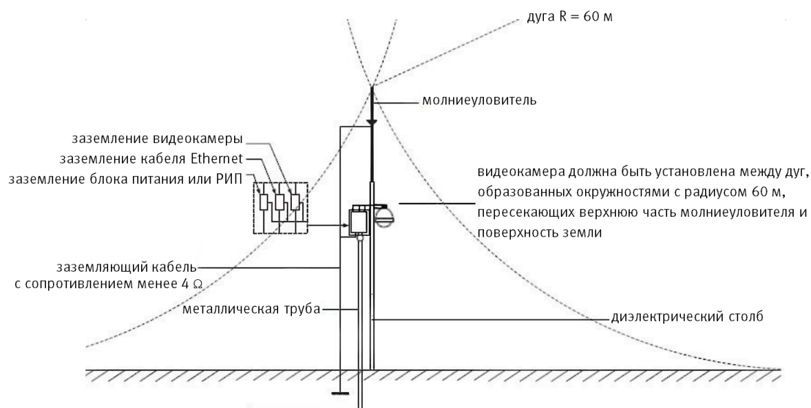
Рисунок 6.13 – Установка молниеотвода
