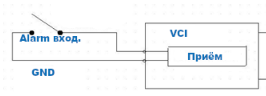
Рисунок 6.12 – Схема подключения тревожного входа
