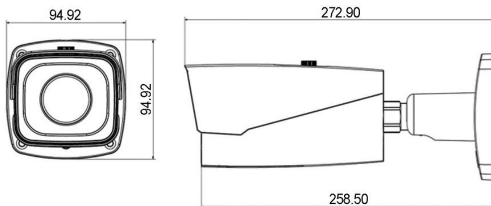
Рисунок 5.1 – Габаритные размеры видеокamеры
