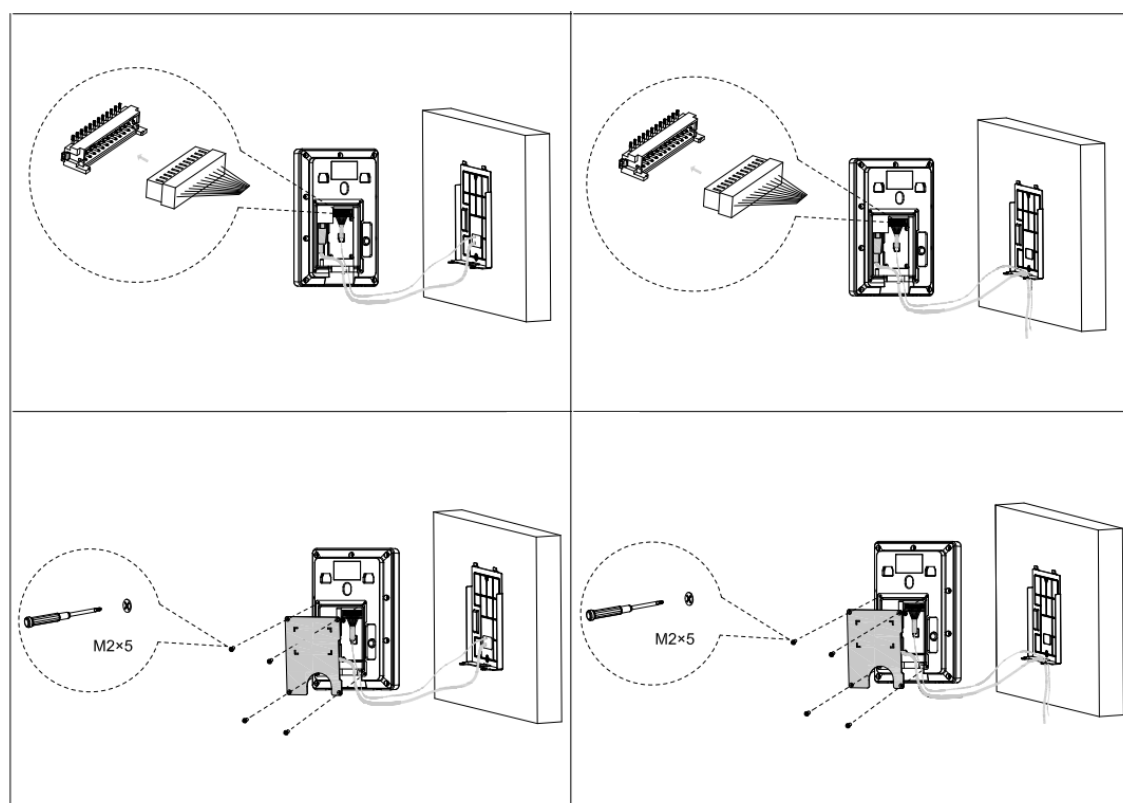
Рисунок 4.7 – Схема установки
