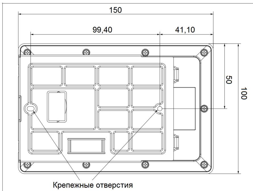
Рисунок 4.5 – Габаритные размеры кронштейна
