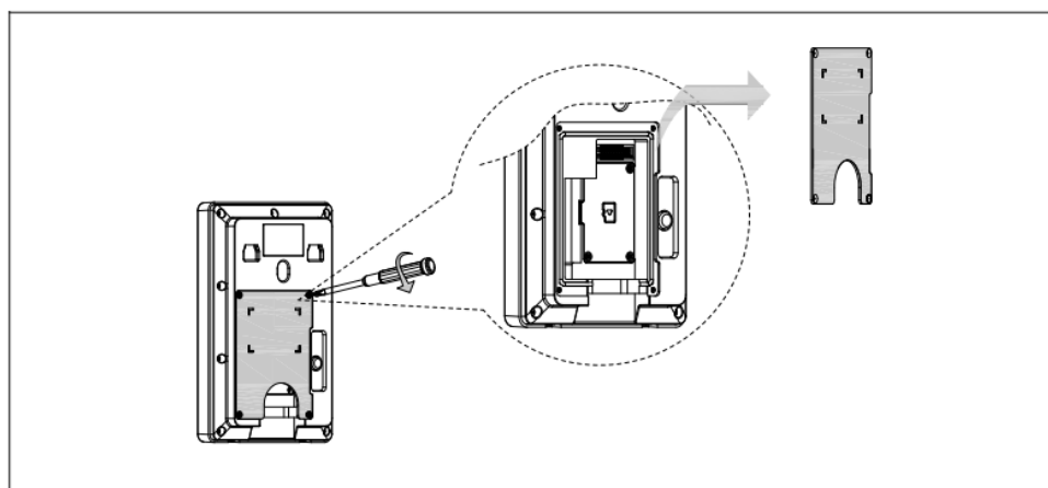
Рисунок 4.3 – Установка карты
