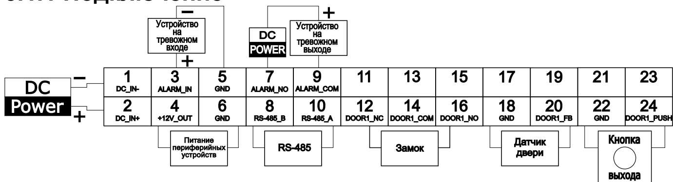
Рисунок 3.2 – Схема
