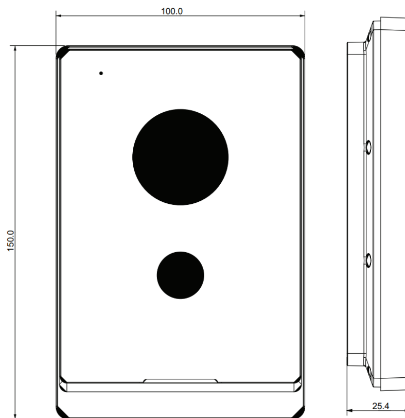
Рисунок 4.1 – Габаритные размеры
