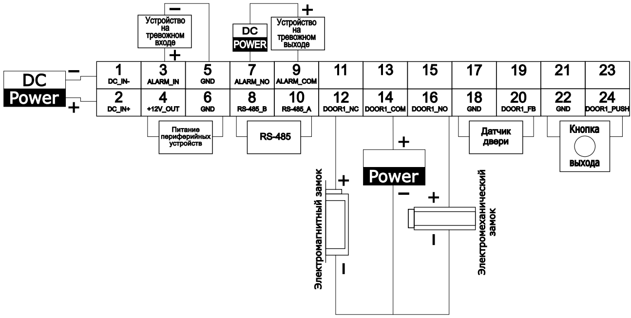
Рисунок 3.3 – Схема подключения. Замок 1
