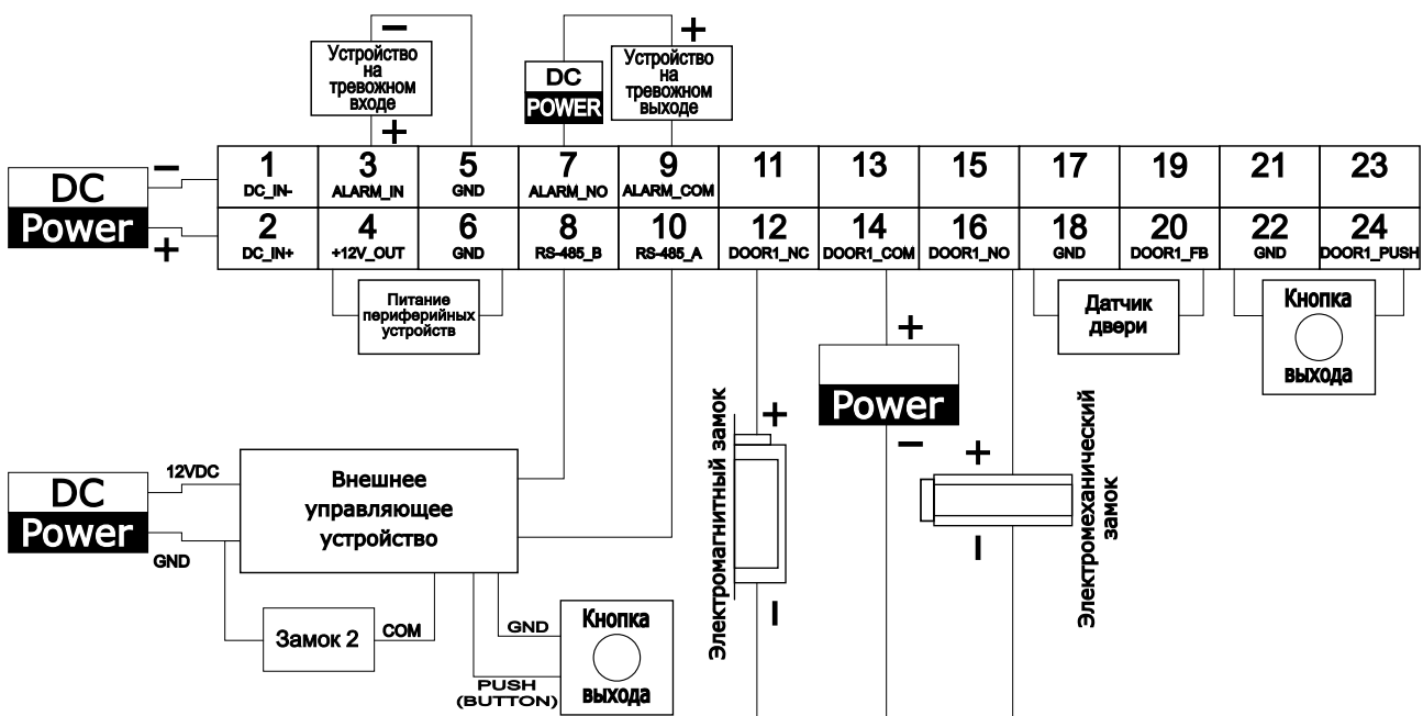
Рисунок 3.4 – Схема подключения. Замок 2
