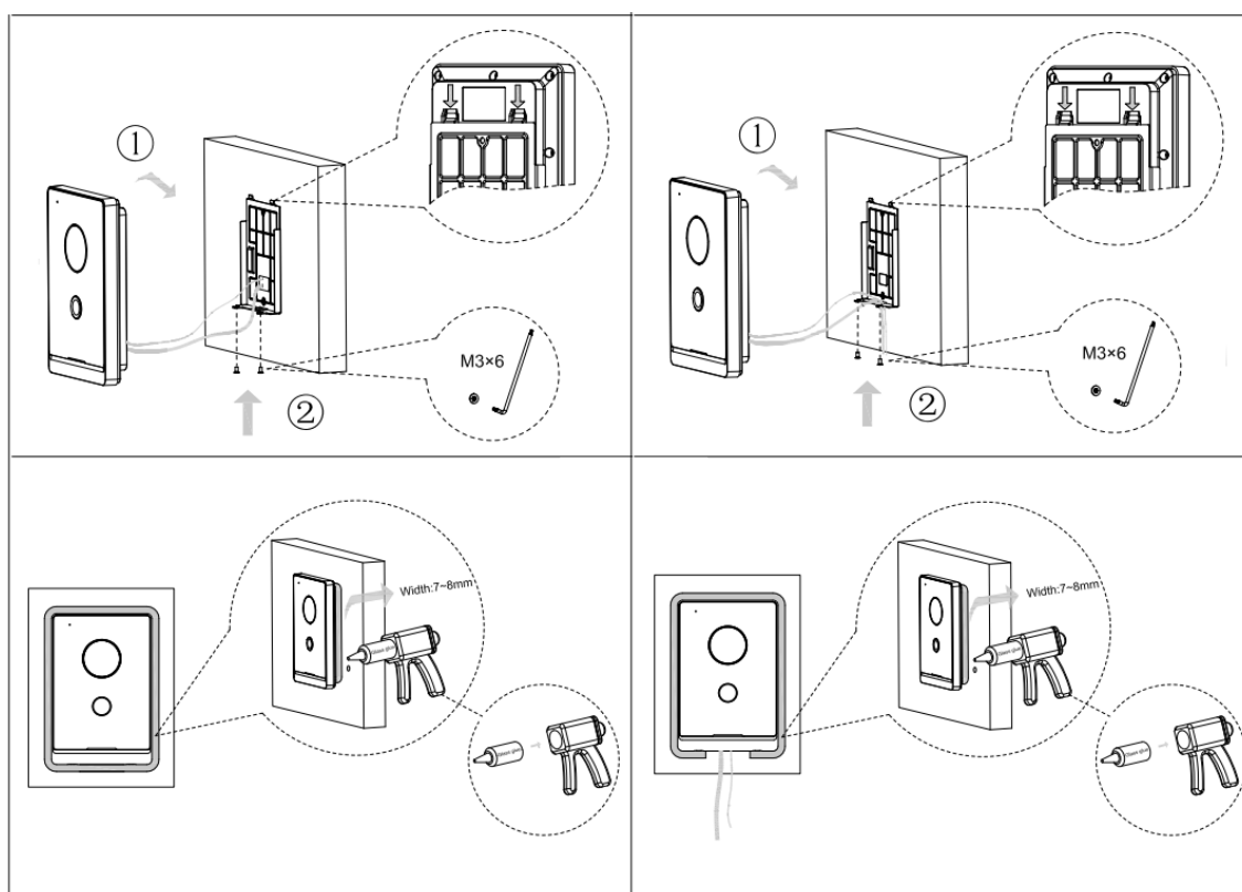
Рисунок 4.8 – Схема установки
