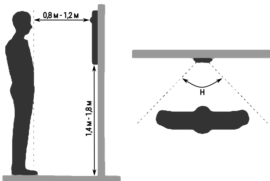
Рисунок 4.2 – Размещение
