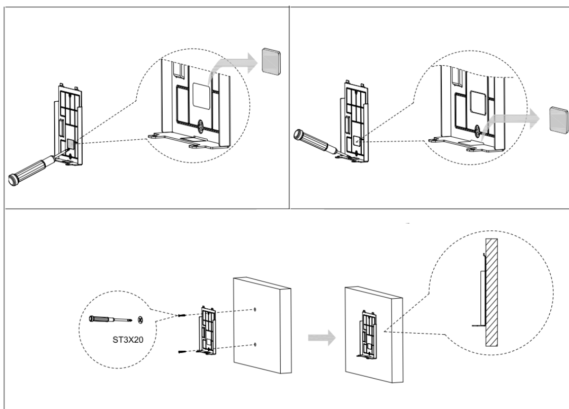
Рисунок 4.6 – Схема установки
