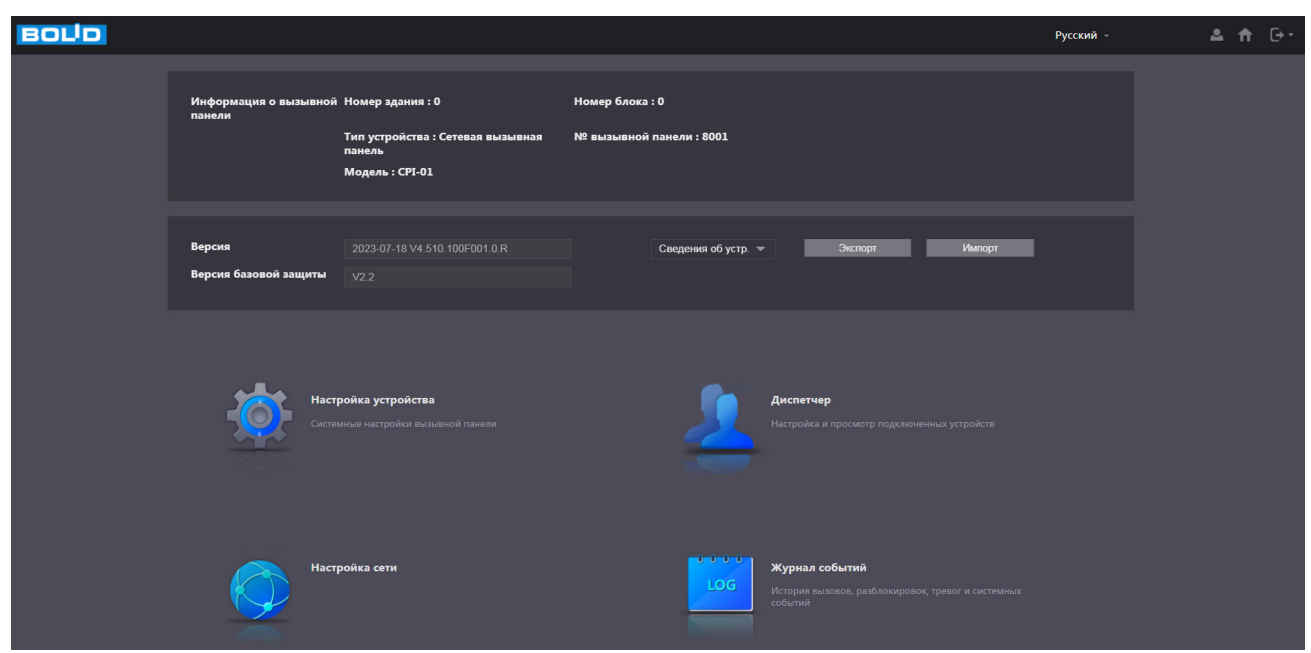
Рисунок 7.1 – Главное меню
