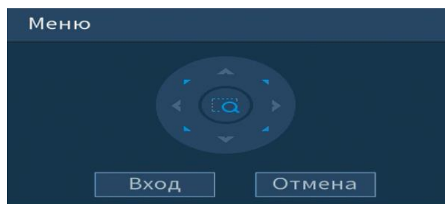
Рисунок 7.3 – Виртуальный джойстик
