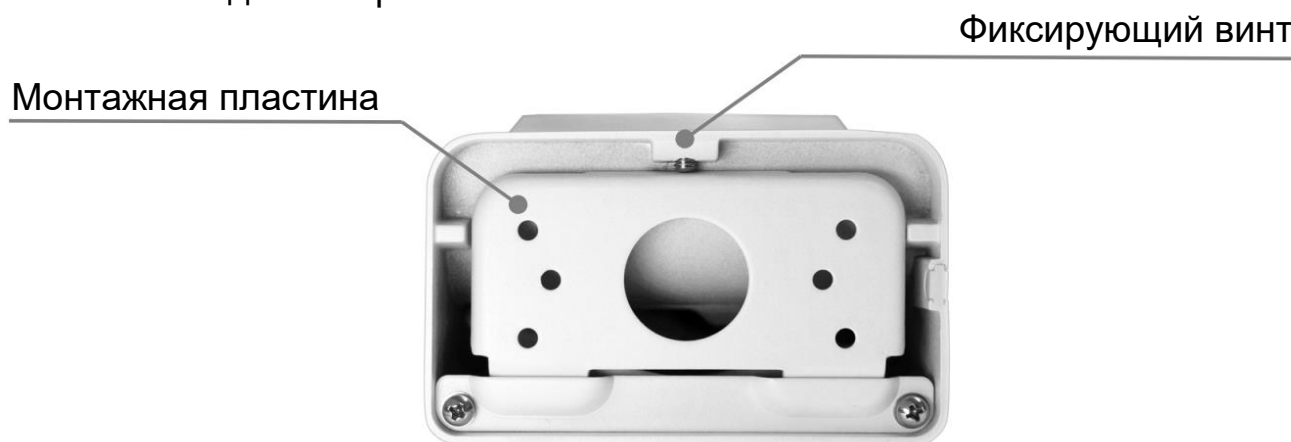
Рисунок 5.5 – Настенный кронштейн
