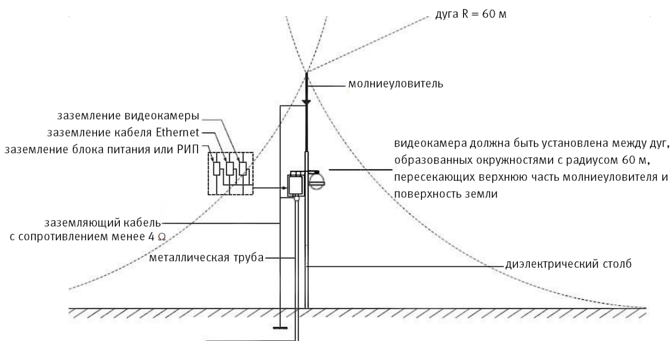
Рисунок 6.5 – Установка молниеотвода
