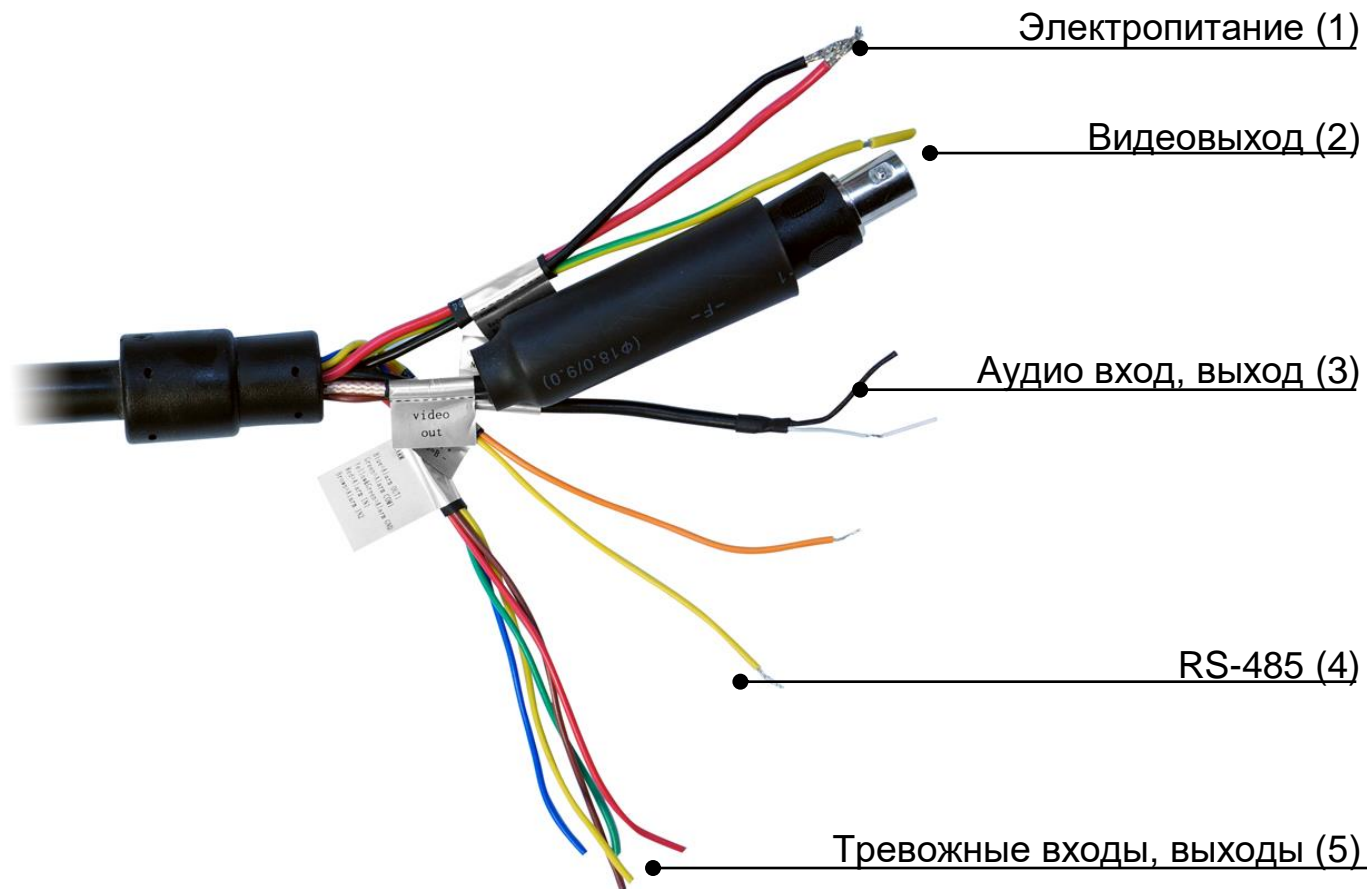
Рисунок 6.1 – Группы концевой раскладки кабеля видеокмеры
