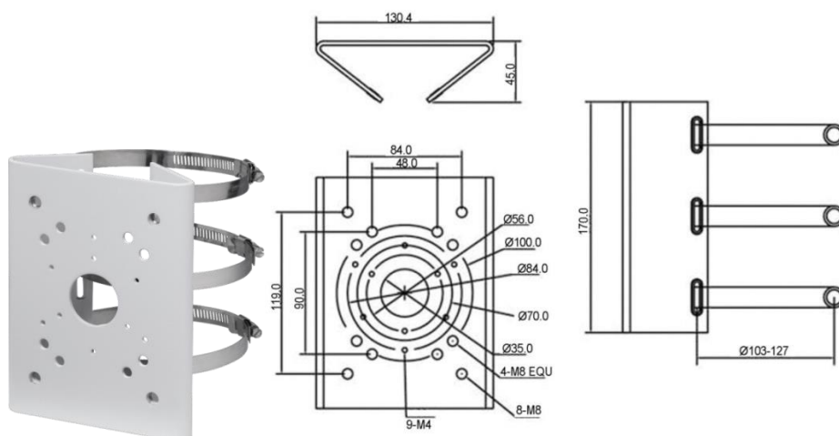
Рисунок 5.10 – Столбовой кронштейн BR-103
