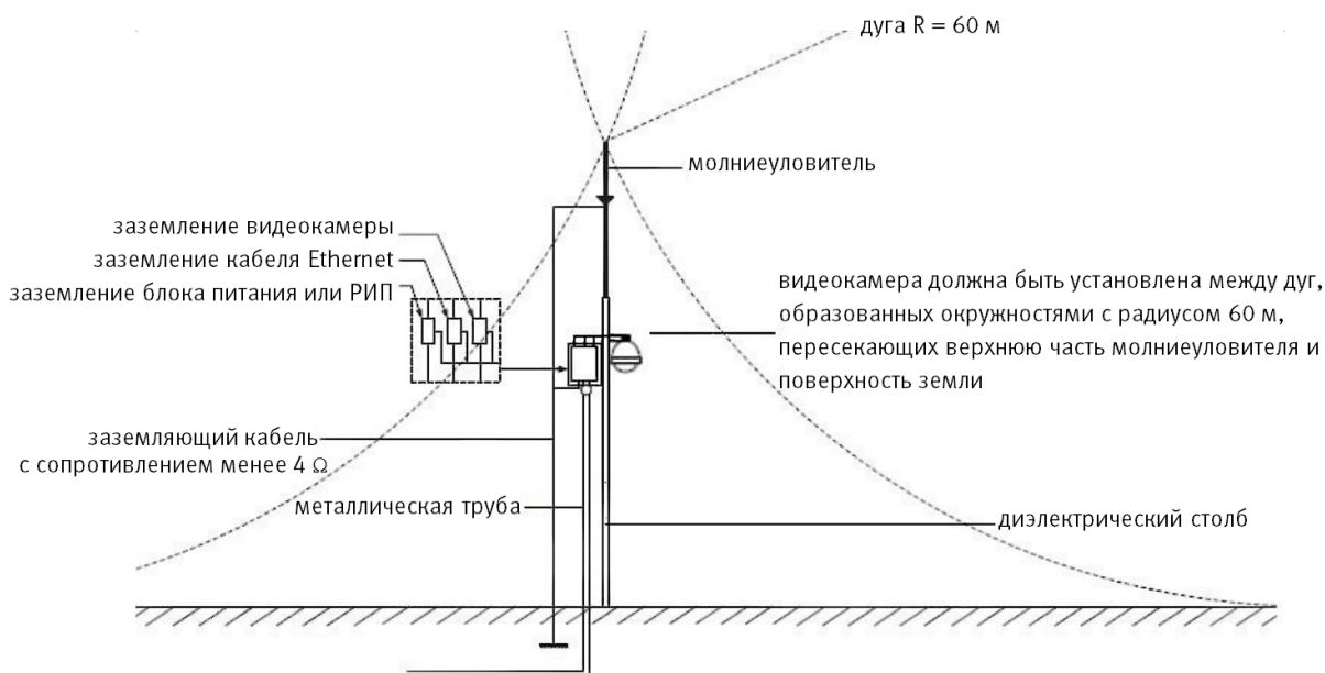
Рисунок 6.6 – Установка молниеотвода
