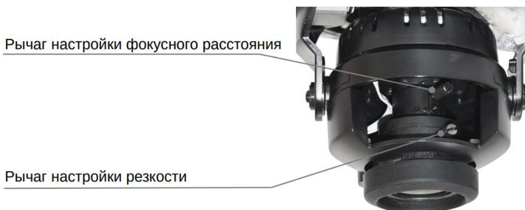
Рисунок 6.4 – Настройка фокусного расстояния и резкости
