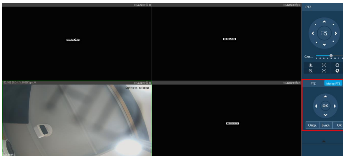
Рисунок 7.1 – Меню PTZ
