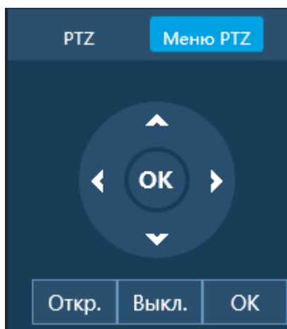
Рисунок 7.2 – Виртуальный джойстик
