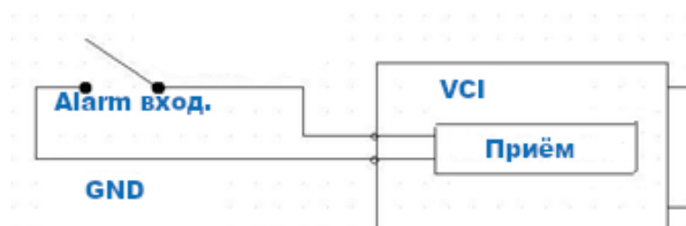
Рисунок 6.12 – Схема подключения тревожного входа
