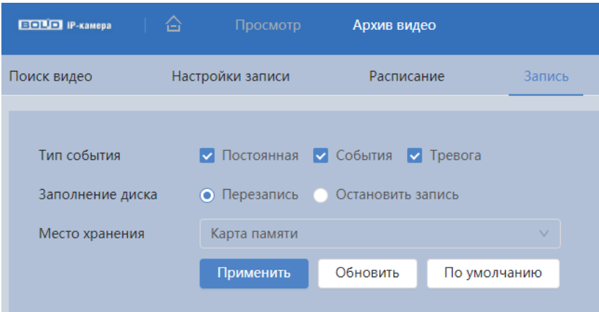
Рисунок 7.90 – Вкладка «Запись»
