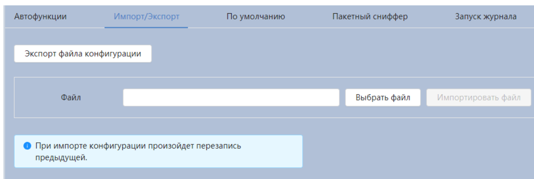
Рисунок 7.78 – Вкладка «Импорт/Экспорт»
