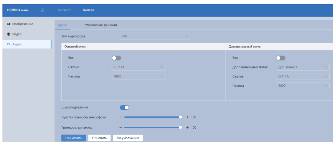
Рисунок 7.48 – Вкладка «Аудио»
