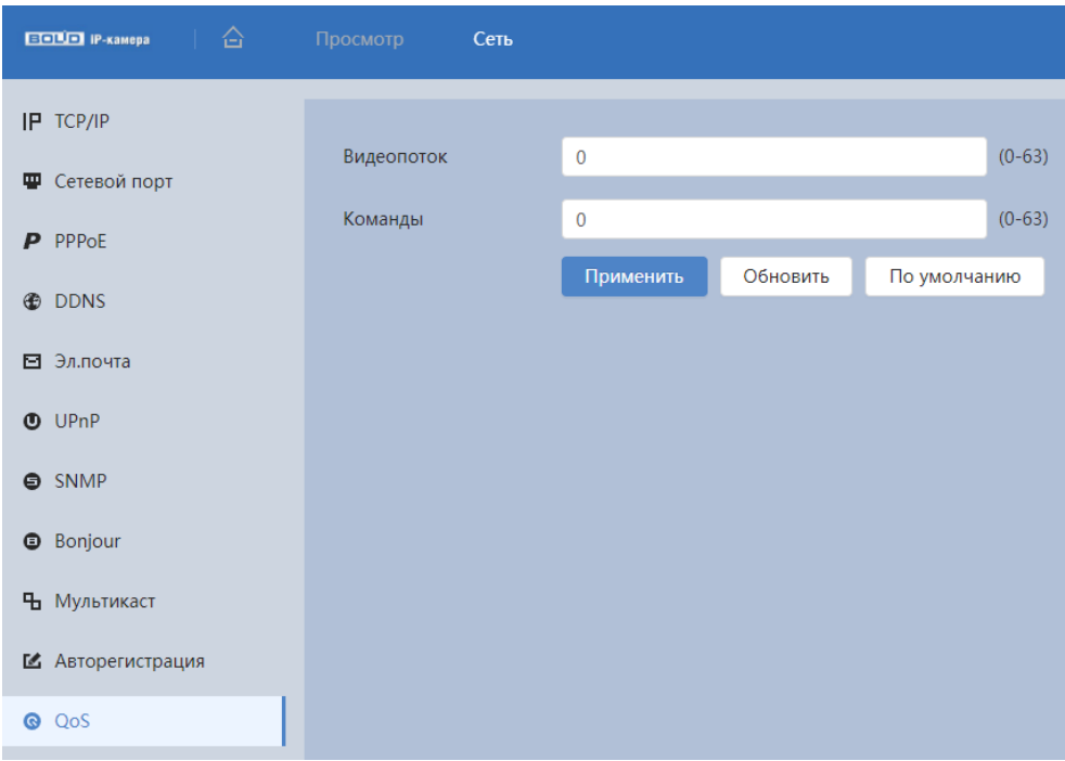
Рисунок 8.17 – Подпункт меню«QoS»
