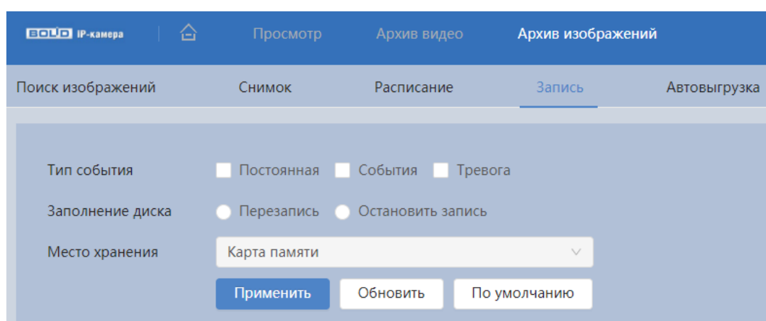
Рисунок 7.97 – Вкладка «Запись»
