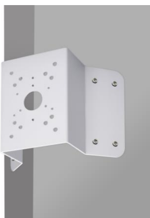
Рисунок 5.11 – Определение точек крепления кронштейна на установочной поверхности
