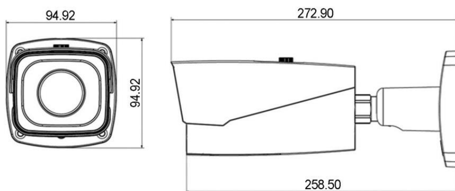
Рисунок 5.1 – Габаритные размеры видеокамеры
