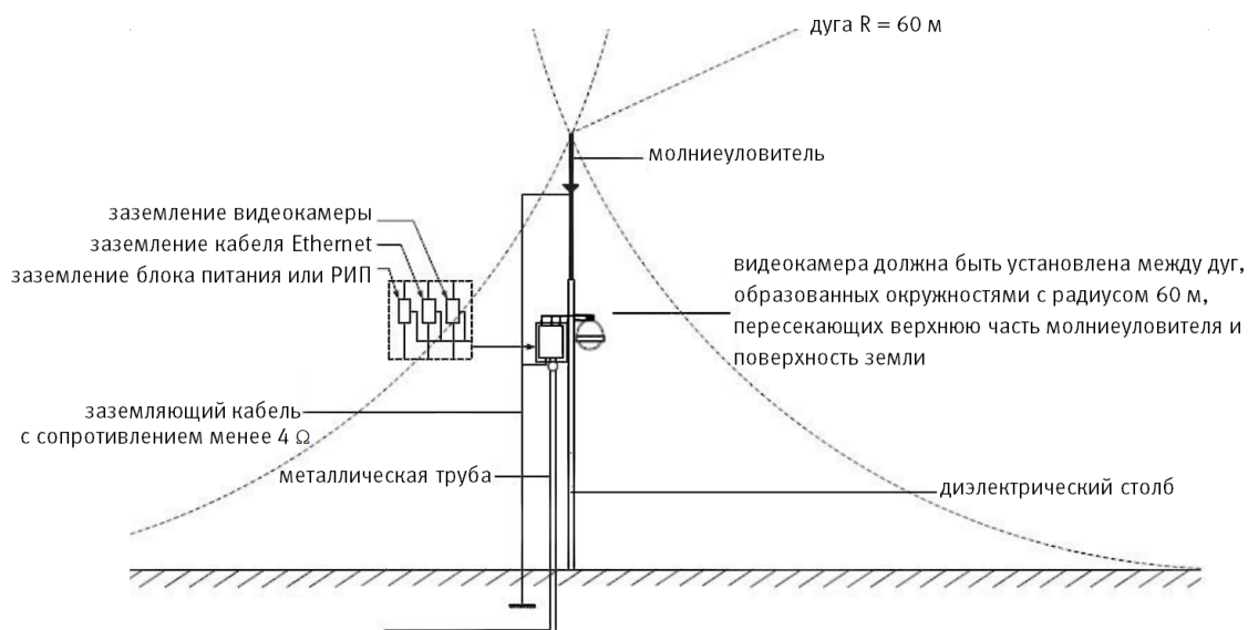
Рисунок 6.14 – Установка молниеотвода
