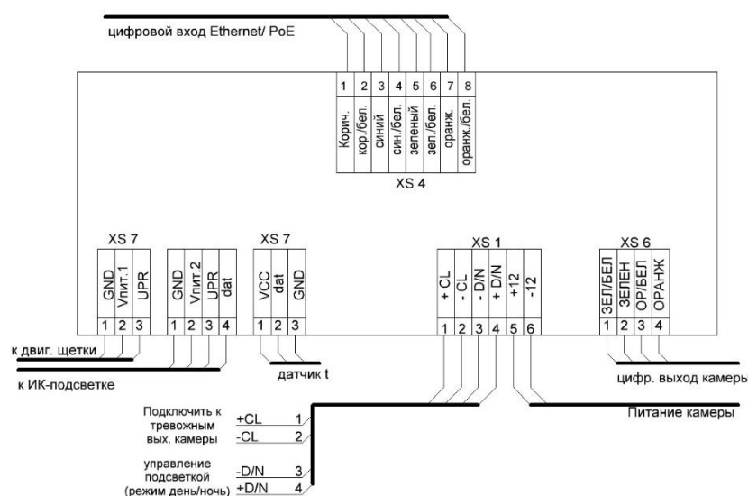
Рисунок 4.3 – Схема подключения термокожуха с напряжением питания по PoE
