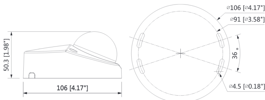
Рисунок 4.1 – Габаритные размеры видеокамеры
