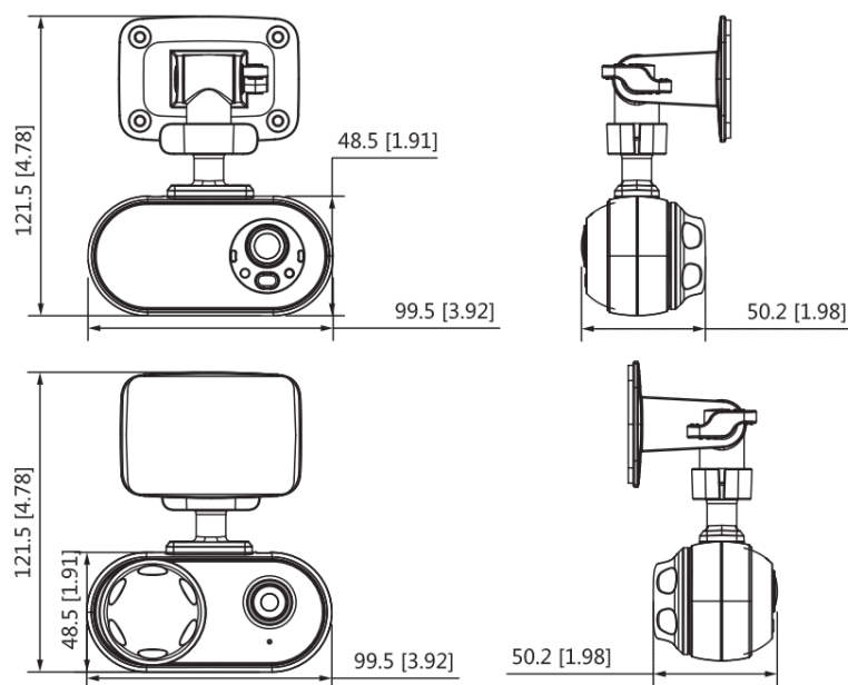
Рисунок 4.1 – Габаритные размеры видеокамеры
