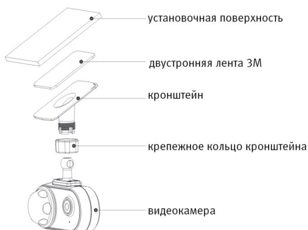
Рисунок 4.2 – Монтаж видеокамеры
