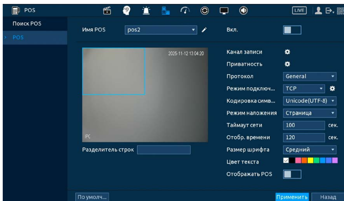
Рисунок 22.2 – POS функция
