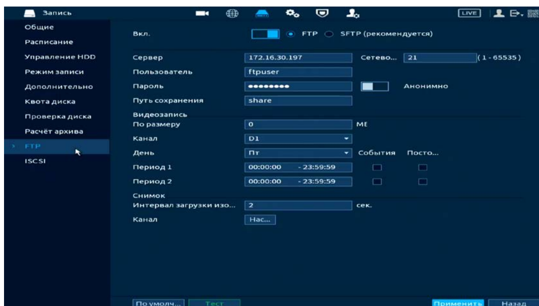
Рисунок 14.29 – Настройка FTP
