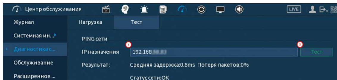
Рисунок 21.10 – Проверка IP-адреса
