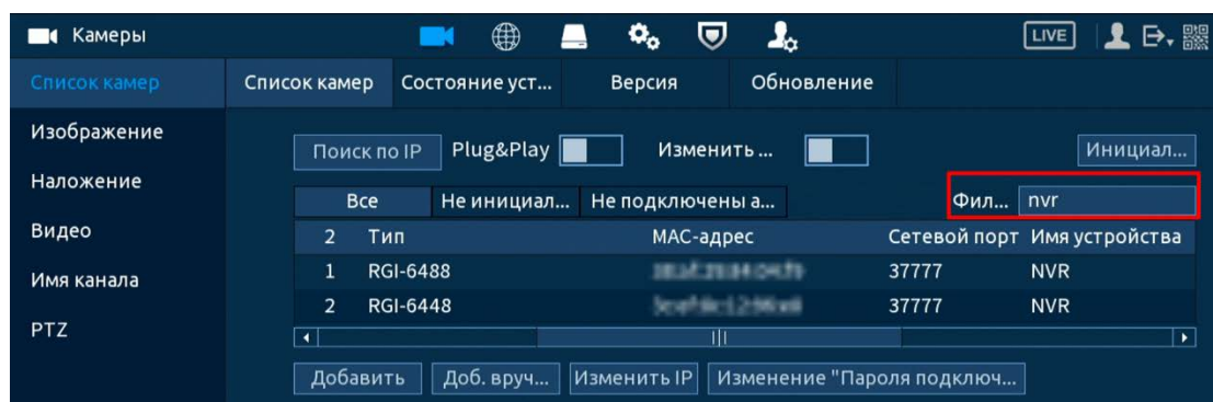
Рисунок 12.8 – Фильтр
