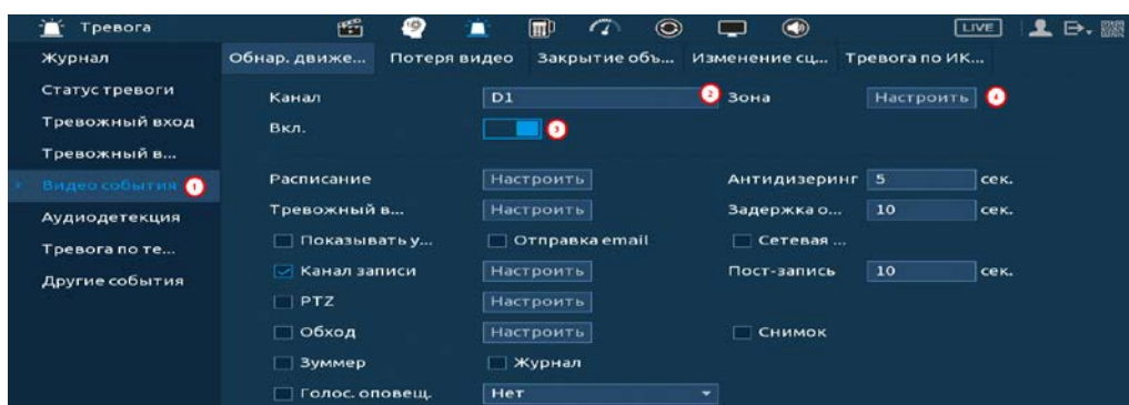
Рисунок 10.8 – Пример настройки
