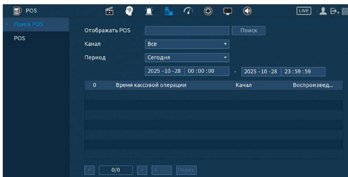
Рисунок 22.1 – POS поиск
