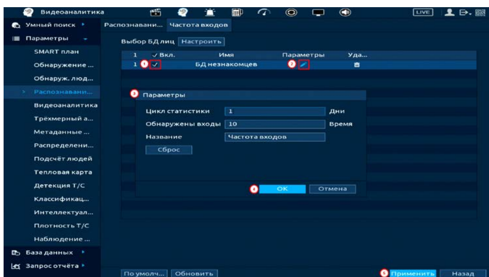
Рисунок 20.31 – Настройка
