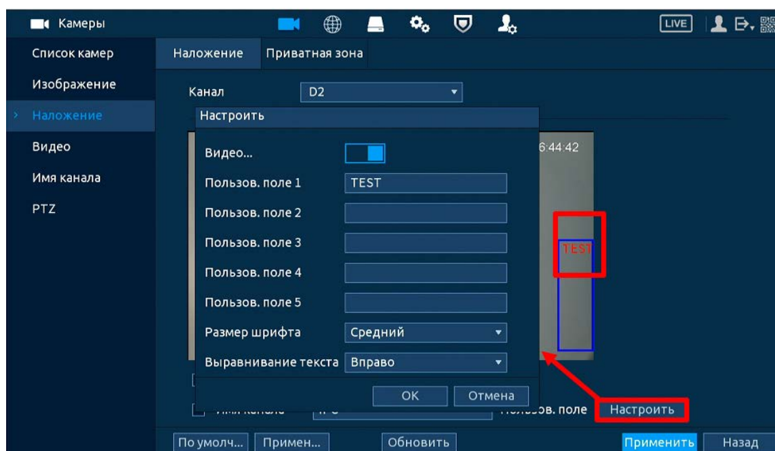
Рисунок 12.34 – Текстовое наложение
