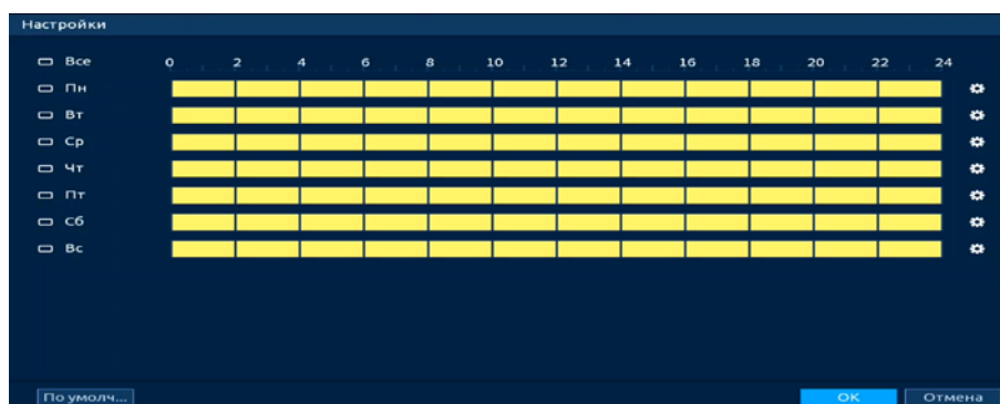
Рисунок 19.38 – Панель расписания
