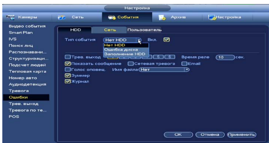
Рисунок 22.8 – Интерфейс настройки оповещения об ошибках HDD
