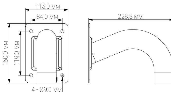
Рисунок 5.5 – Габаритные размеры настенного кронштейна
