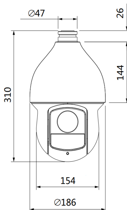
Рисунок 5.1 – Габаритные размеры видеокamеры
