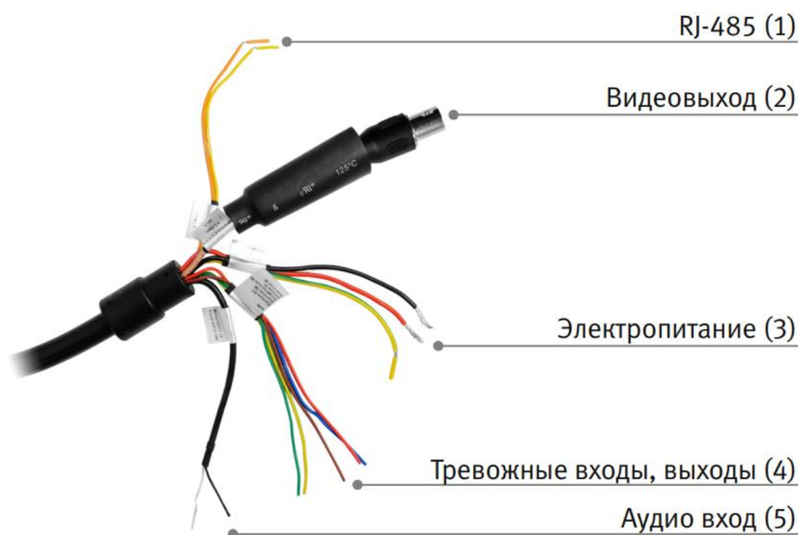
Рисунок 6.1 – Группы концевой раскладки кабеля видеоканеры
