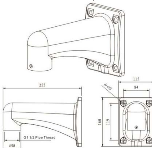
Рисунок 4.7 – Габаритные размеры кронштейна
