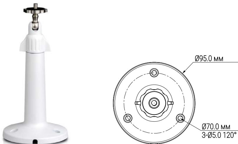
Рисунок 4.11 – Кронштейн BR-101
