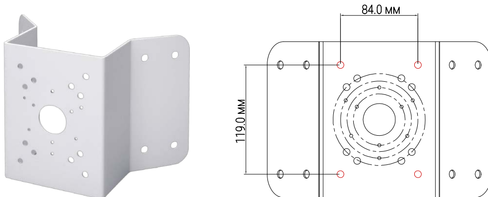
Рисунок 4.6 – Угловой кронштейн BR-102
