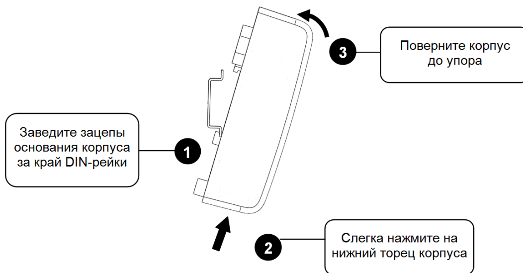
Рисунок 2.4 Монтаж на DIN-рейку
