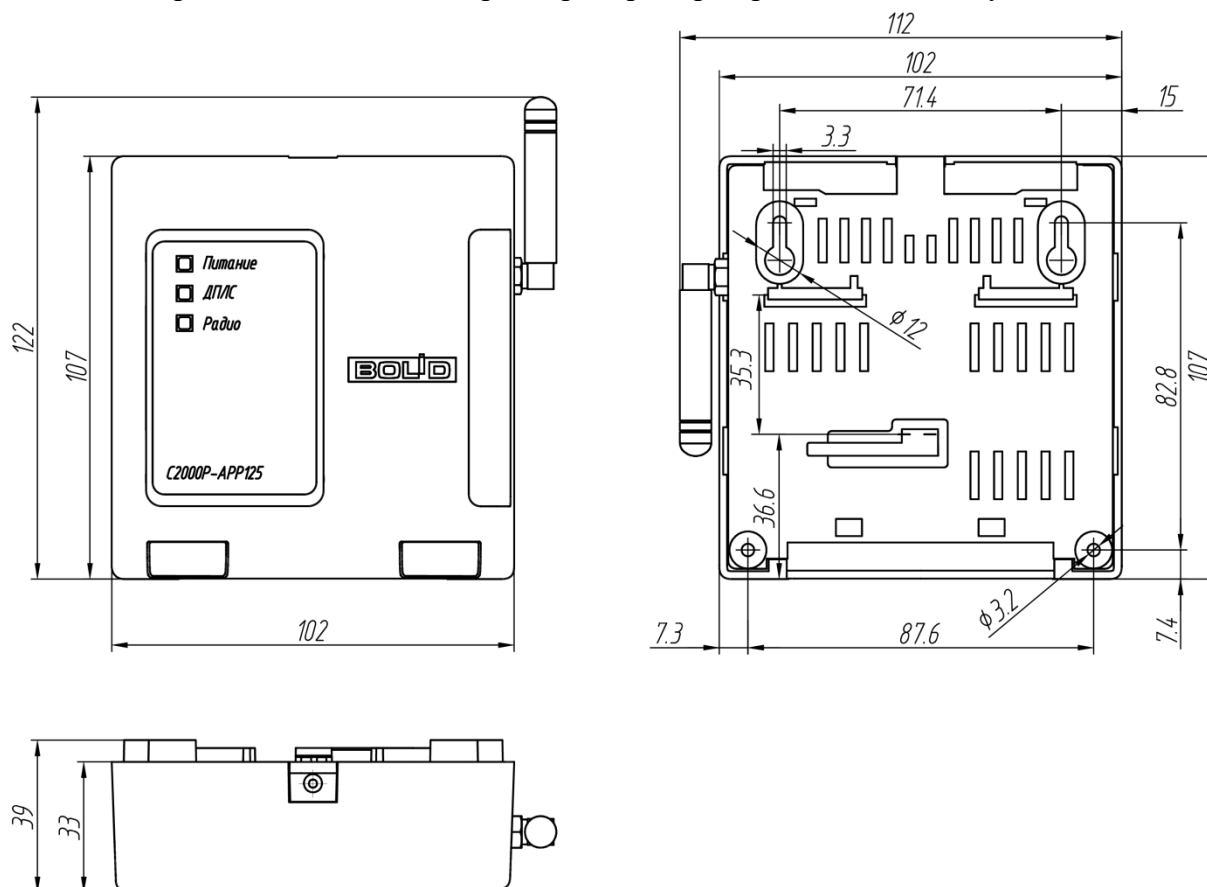
Рисунок 2.3 Габаритные и монтажные размеры
