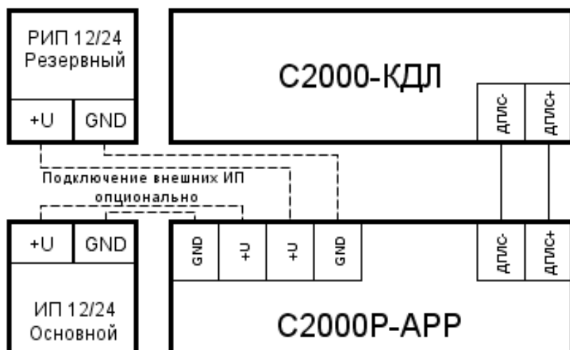
Рисунок 2.5 Схема подключения радиорасширителя
