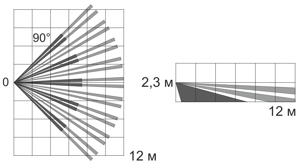
Рисунок 2.5 Зона обнаружения
