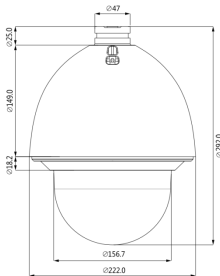
Рисунок 5.1 – Габаритные размеры видеокamеры (мм)
