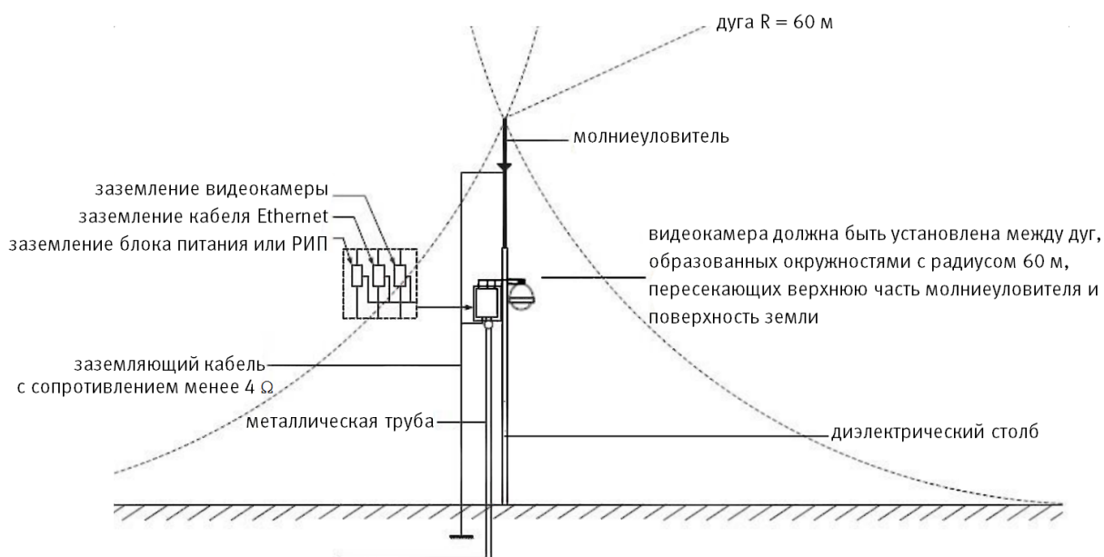
Рисунок 6.13 – Установка молниеотвода
