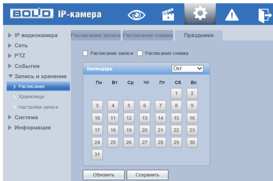
Рисунок 7.126 – Вкладка «Праздники»
