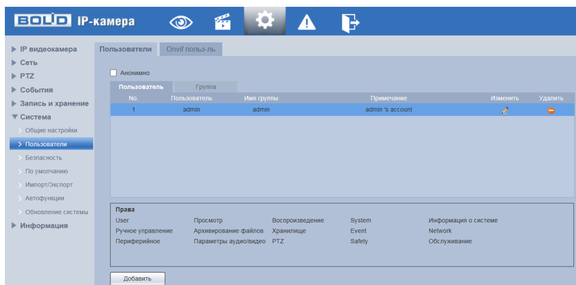
Рисунок 7.136 – Вкладка «Пользователи»
