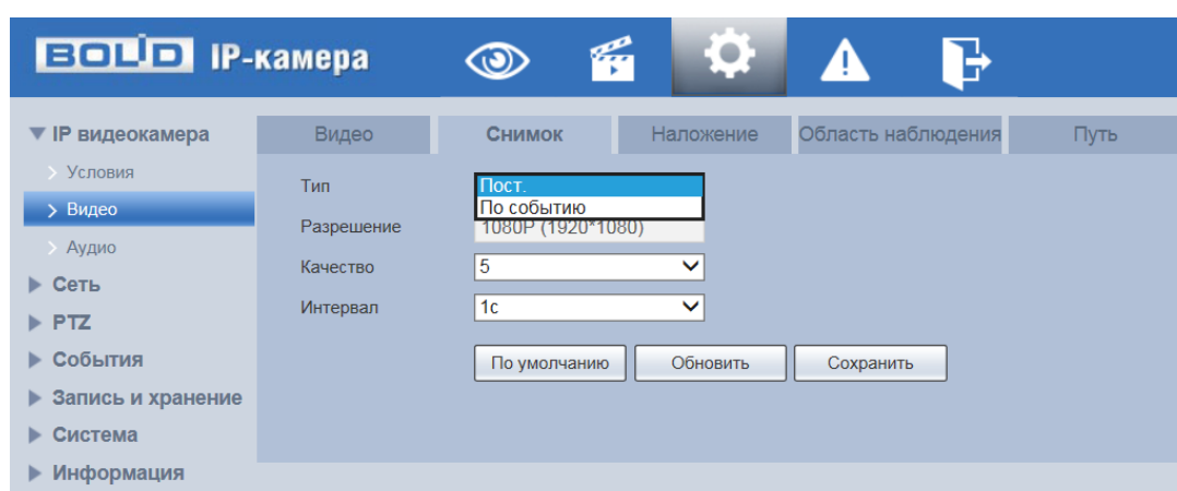
Рисунок 7.44 – Вкладка «Снимок»
