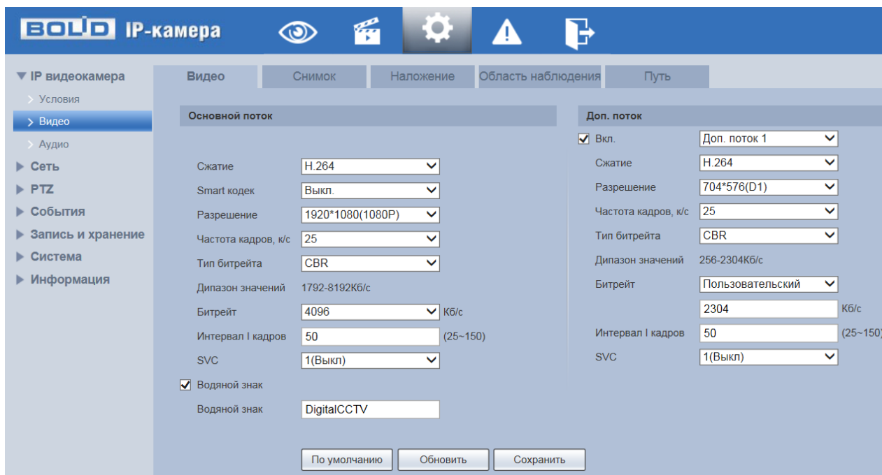
Рисунок 7.43 – Вкладка «Видео»
