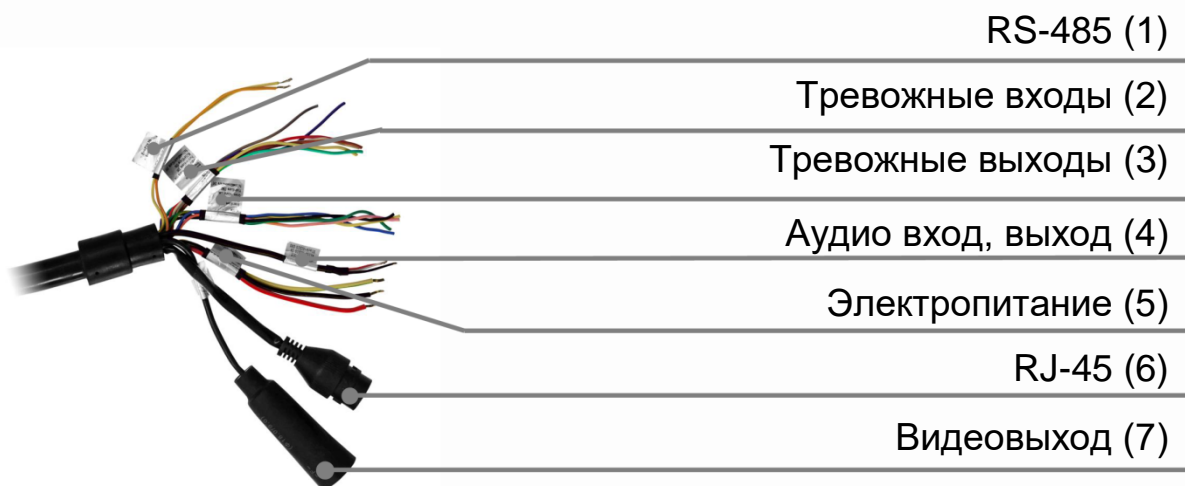
Рисунок 6.1 – Группы концевой раскладки кабеля видеокмеры
