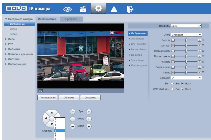
Рисунок 7.31 – Вкладка «Изображение»
