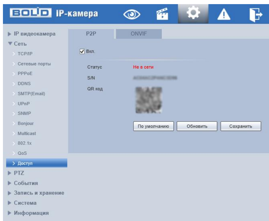
Рисунок 7.73 – Вкладка «P2P»
