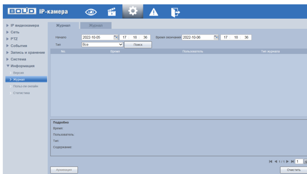
Рисунок 7.152 – Вкладка «Журнал»
