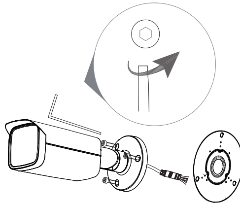
Рисунок 4.4 – Монтаж
