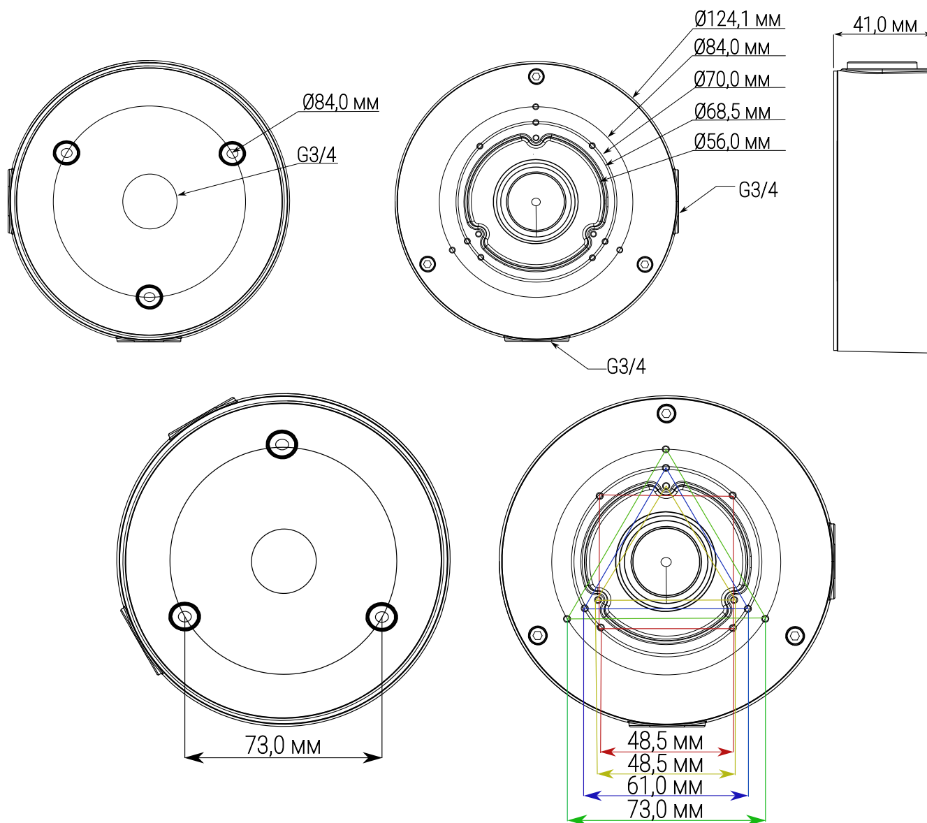
Рисунок 4.1 – Габаритные размеры
