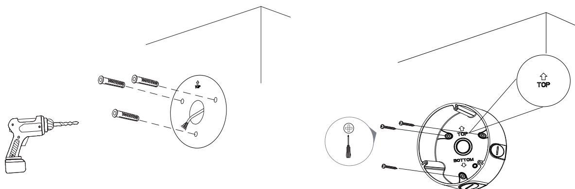
Рисунок 4.3 – Монтаж
