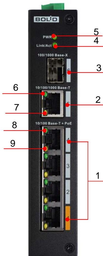
Рисунок 4.2 – Передняя панель
