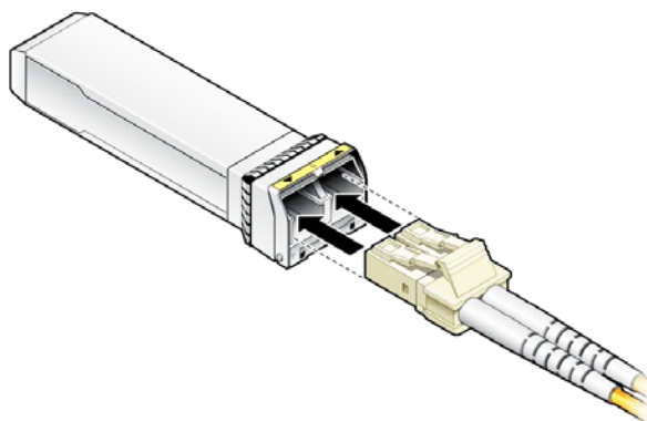
Рисунок 5.5 – Подключения кабеля
