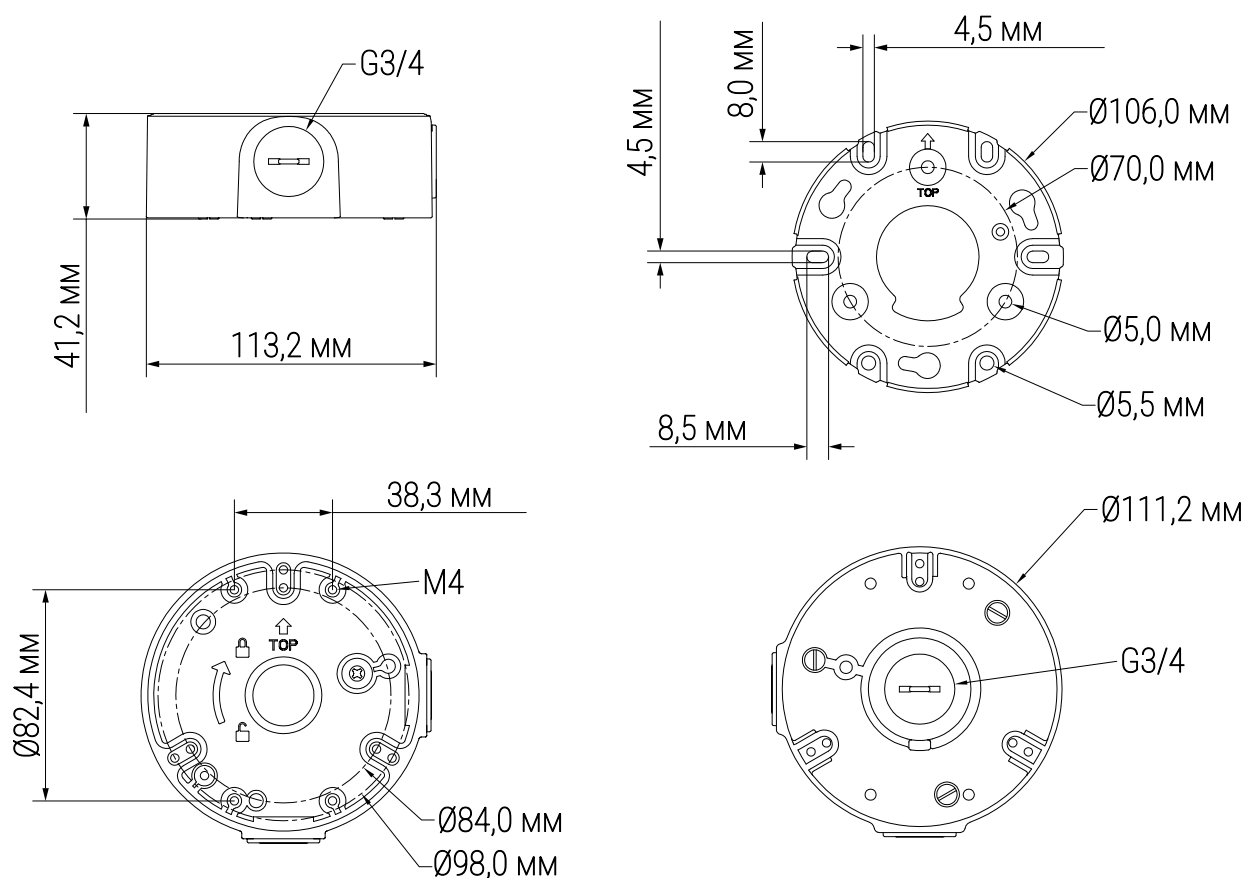
Рисунок 4. 1 – Габаритные размеры
