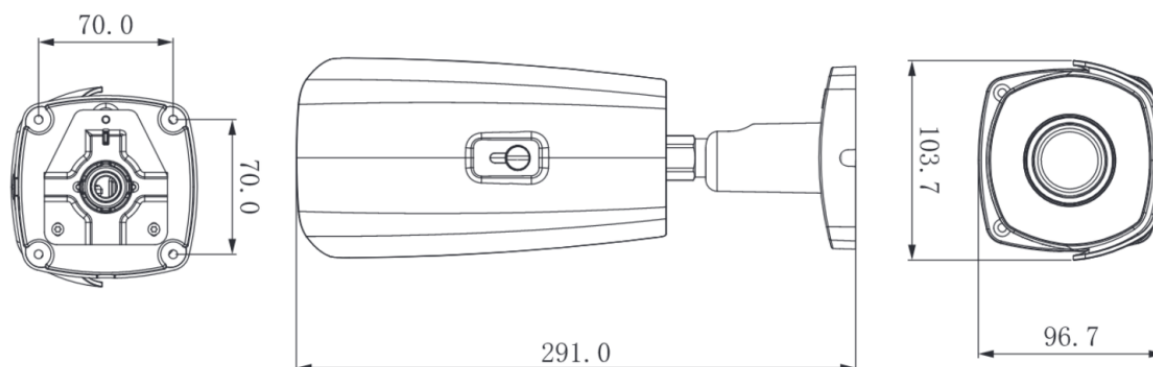
Рисунок 4.3 – Габаритные размеры видеокамеры
