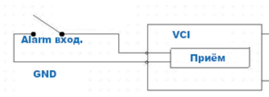
Рисунок 6.12 – Схема подключения тревожного входа
