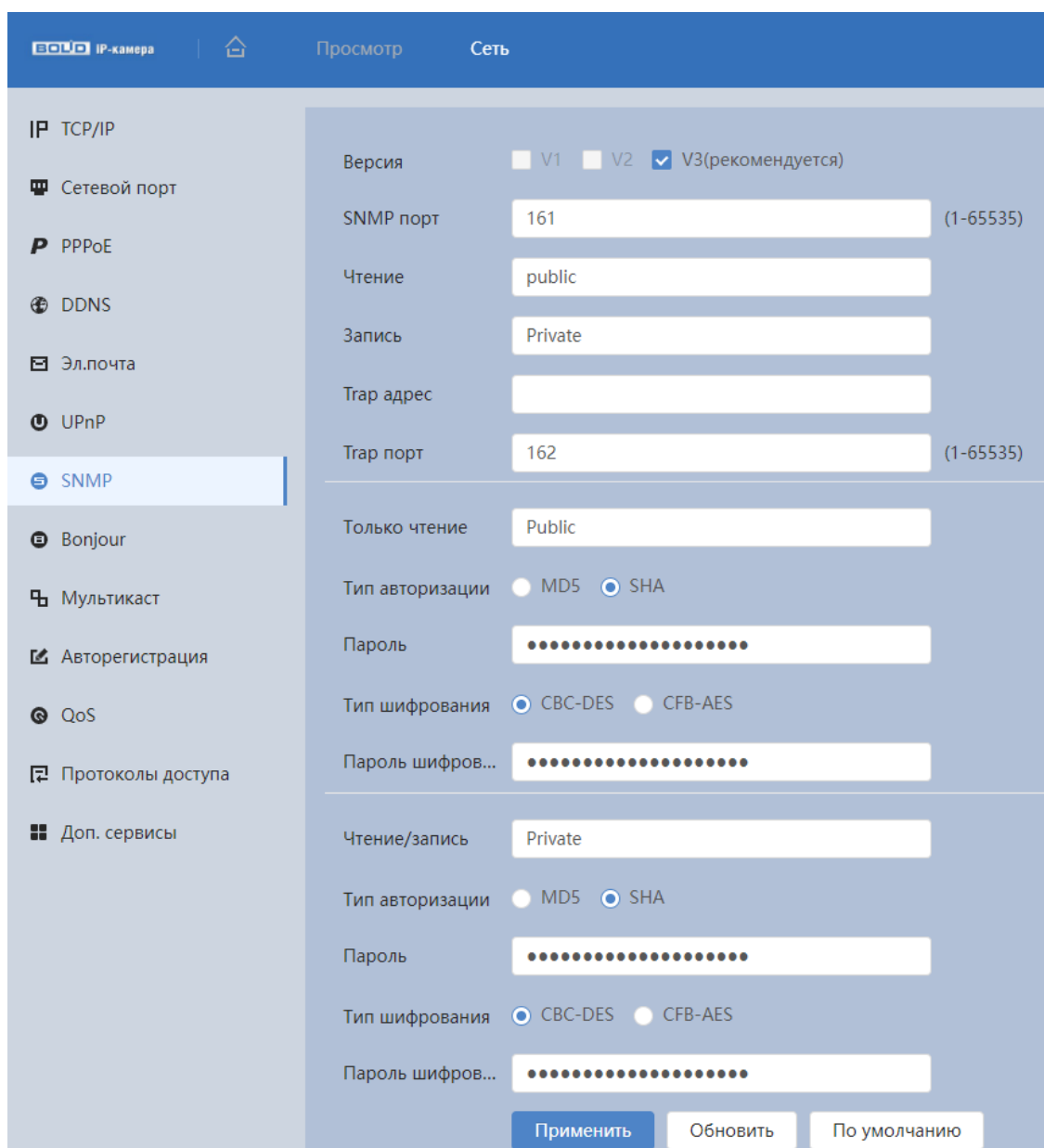
Рисунок 8.13 – Подпункт меню «SNMP»
