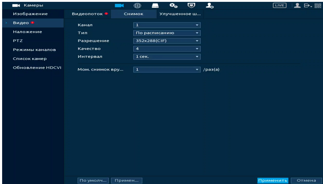
Рисунок 11.6 – Настройка снимка
