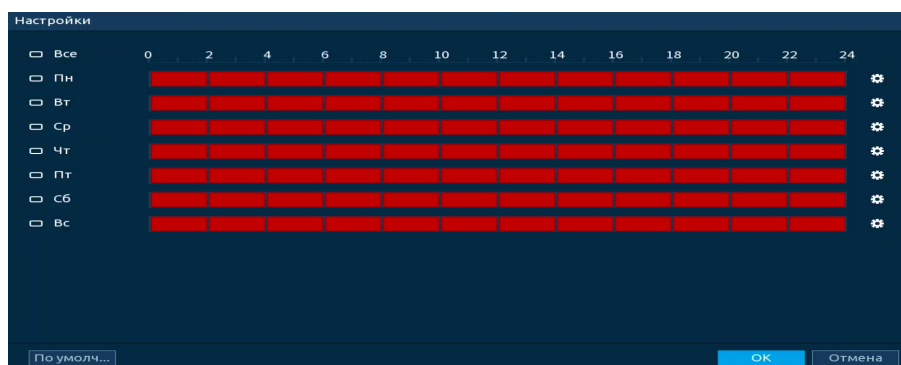
Рисунок 18.11 – Панель расписания
