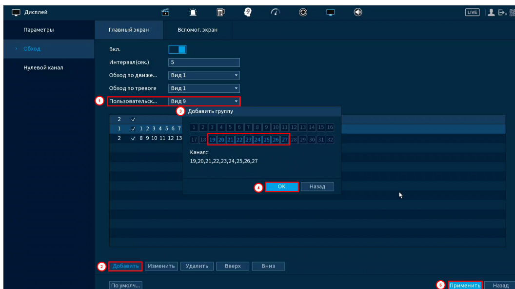
Рисунок 23.10 – Добавление группы
