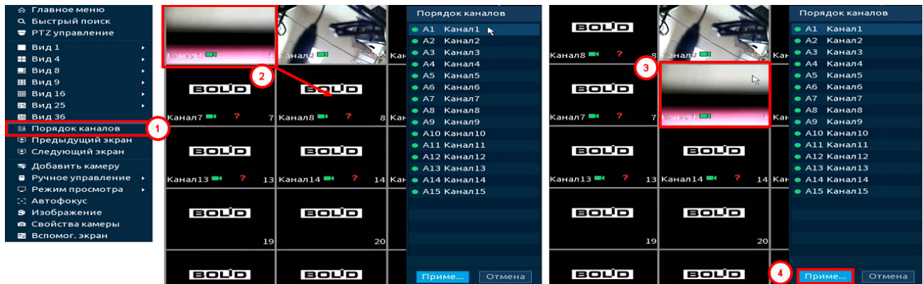
Рисунок 7.8 – Изменение раскладки
