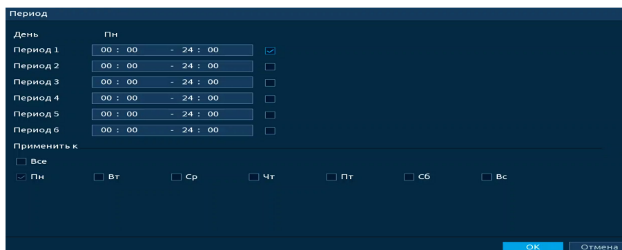
Рисунок 18.12 – Расписание
