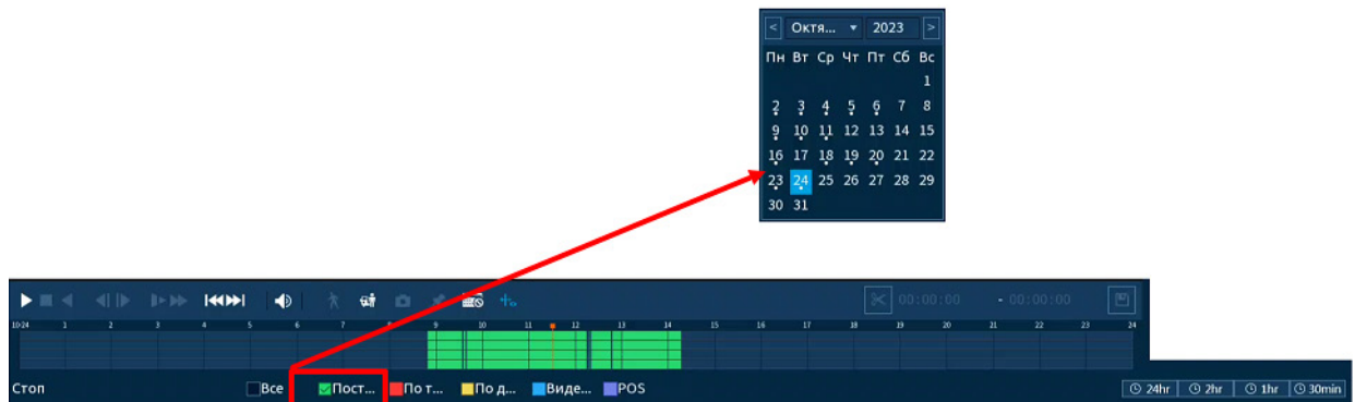
Рисунок 17.5 – Шкала времени
