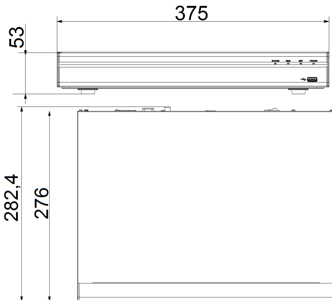
Рисунок 4.1 – Габаритные размеры видеорегистратора
