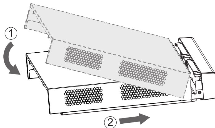
Рисунок 4.6 – Установка жесткого диска
