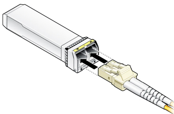
Рисунок 5.5 – Подключения кабеля
