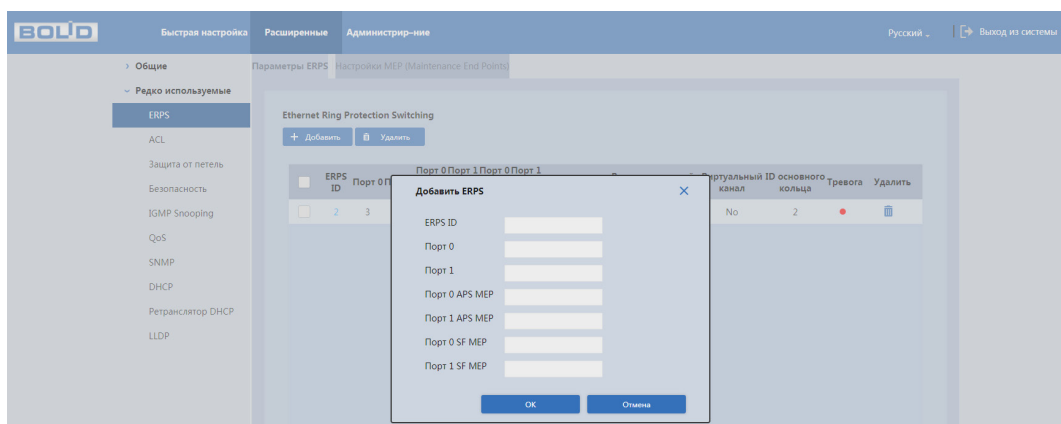
Рисунок 11.7 – Добавление ERPS
