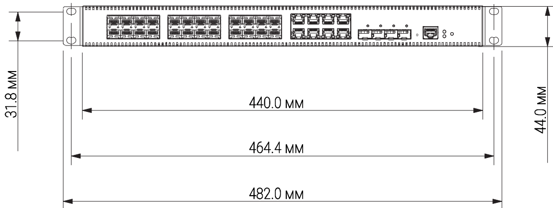
Рисунок 5.2 – Габаритные размеры
