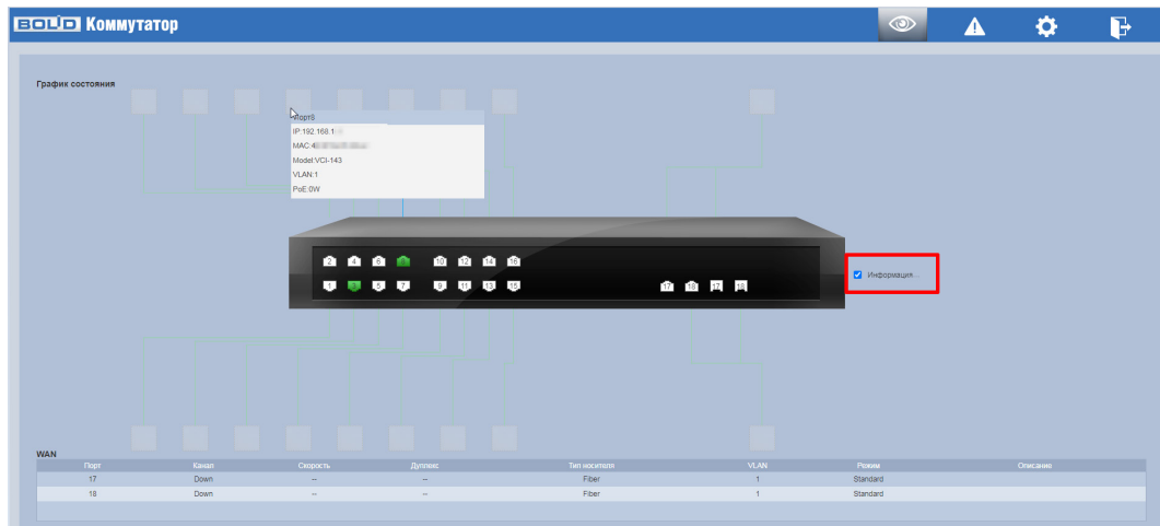
Рисунок 7.3 – Графическая панель
