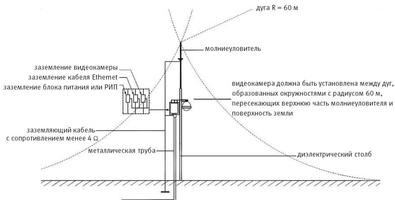
Рисунок 6.14 – Установка молниеотвода
