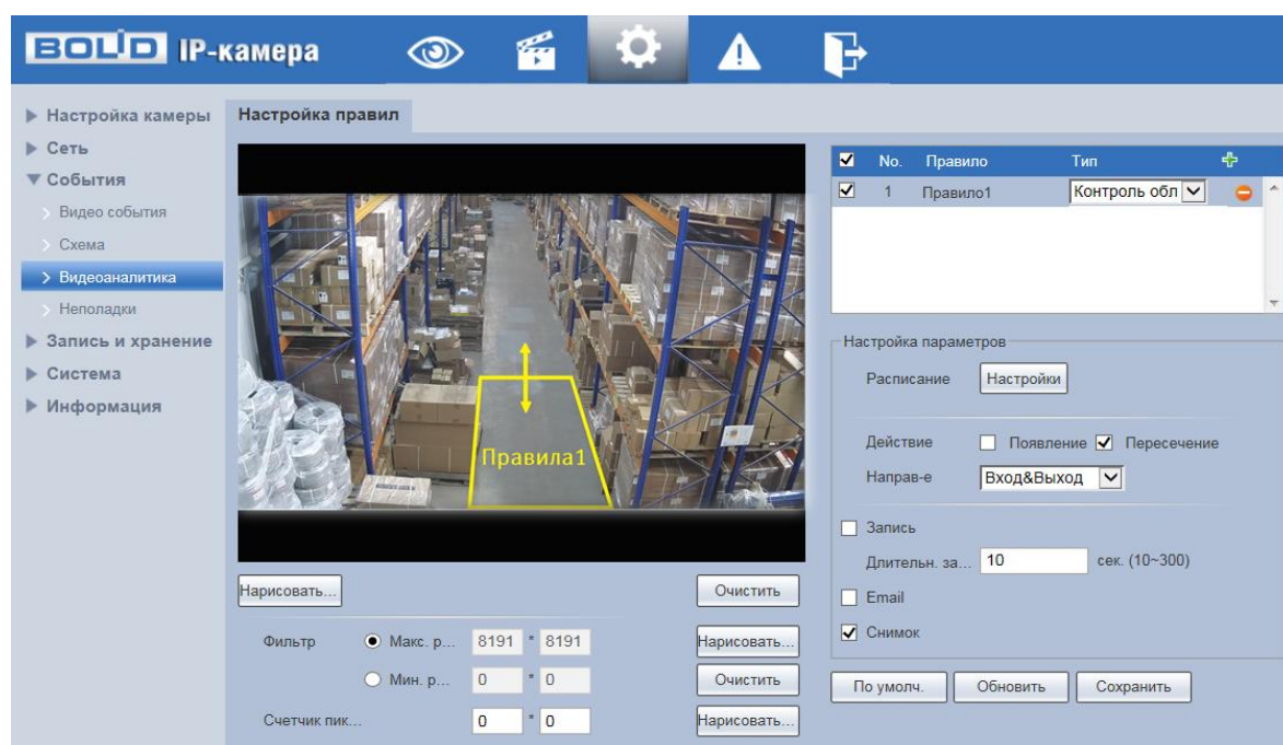
Рисунок 7.77 – Создание правила видеоаналитики «Контроль области»
