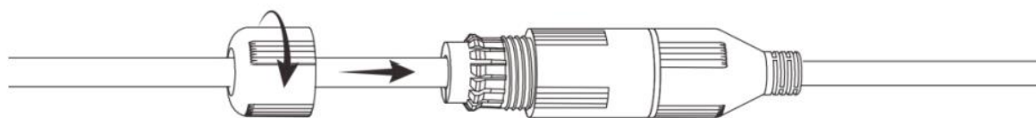
Рисунок 6.10 – Совмещение колпачка с основанием герметичной кабельной муфты
