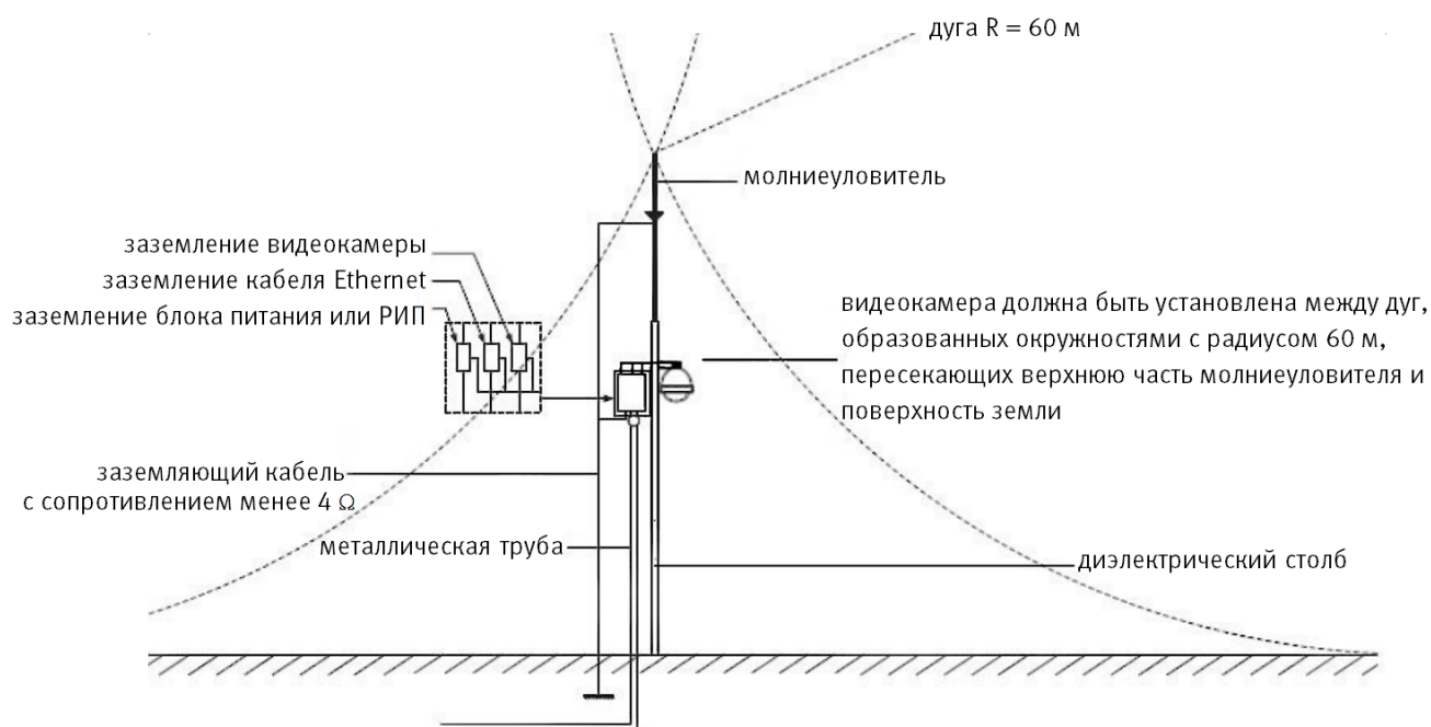
Рисунок 6.14 – Установка молниеотвода
