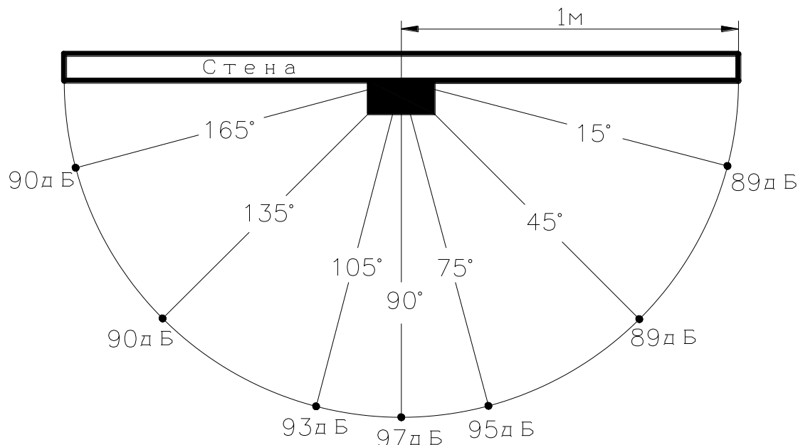
Рисунок 2.2.3.2 Диаграмма направленности ОПЗ
