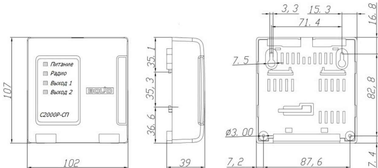
Рисунок 2.3 Монтажные размеры
